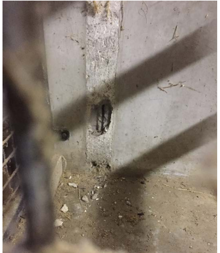
nr: 30 toelichting: geroeste wapening in beton plaats: Interieur dierenverblijf
