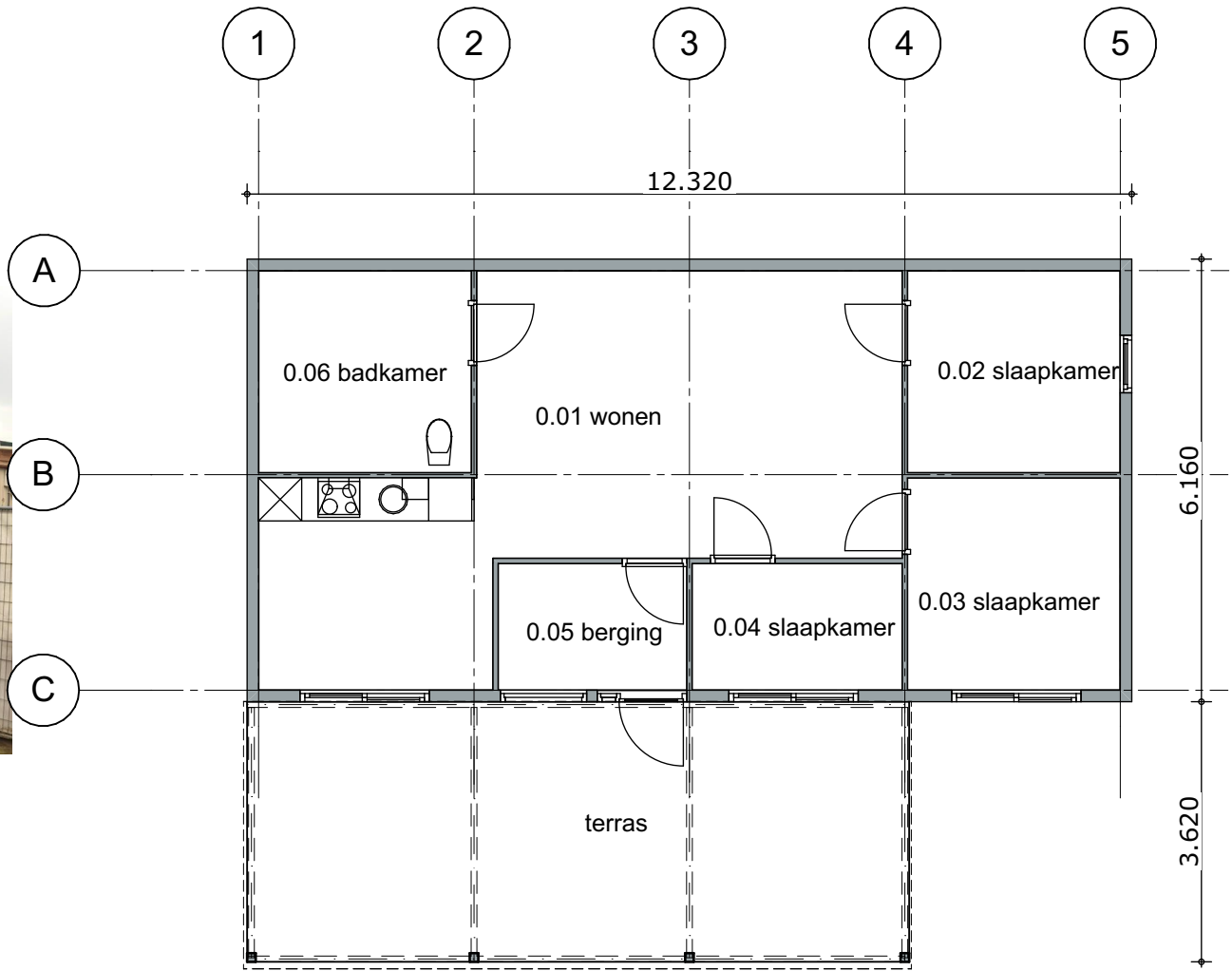
PLATTEGROND
