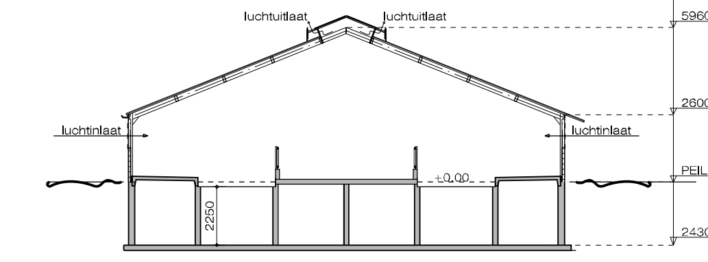
doorsnede F-F
