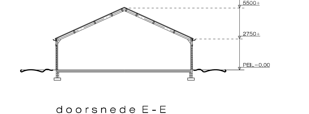
doorsnede E-E
