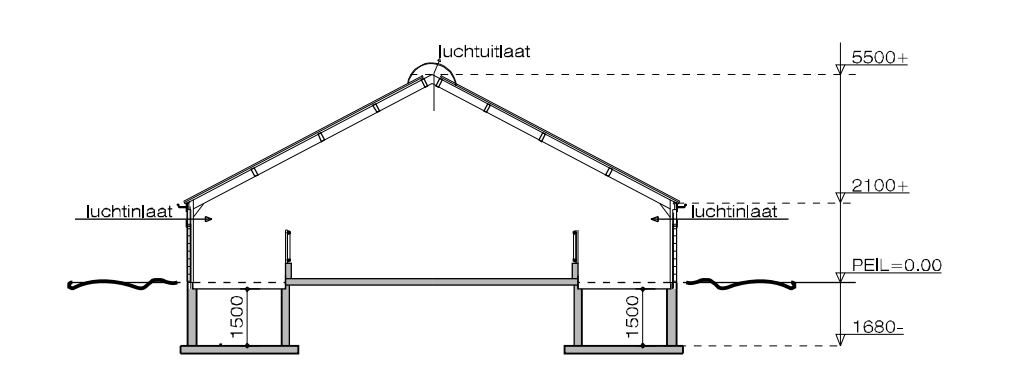
doorsnede C-C
