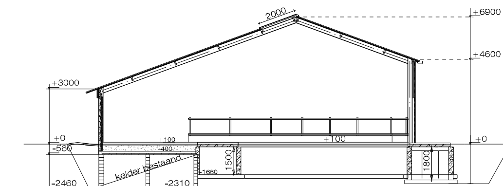
doorsnede B2
