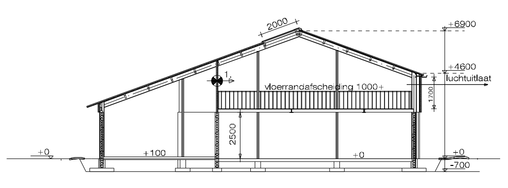
doorsnede B1
