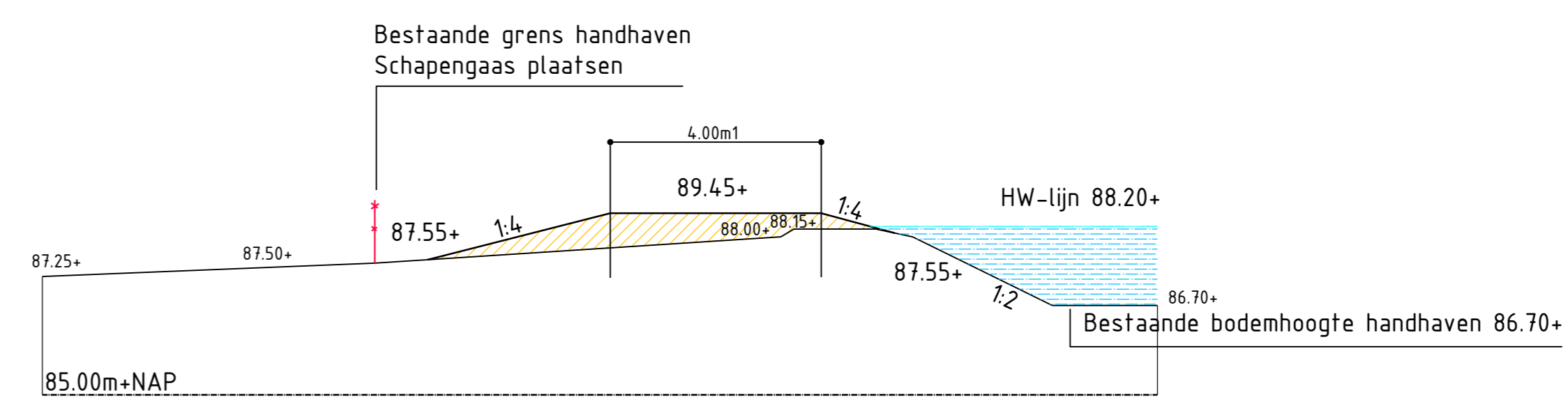
Profiel A-A buffer RESL22 Schaal 1:100
