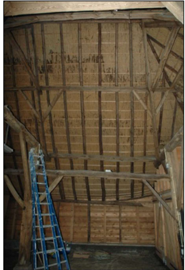
Afb. @ [LB]: Binnenkant van het voorste dakvlak met het A-vormige bovenjuk.
