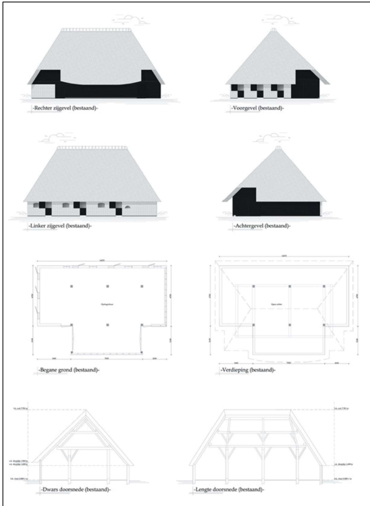
Afb. @: De kleine schuur getekend in de bestaande toestand. Gevels, plattegronden en doorsneden genomen uit de bouwtekening (afb. @, bijlage). [Mathijssen Ontwerp / Veerman Bouwhistorie]
