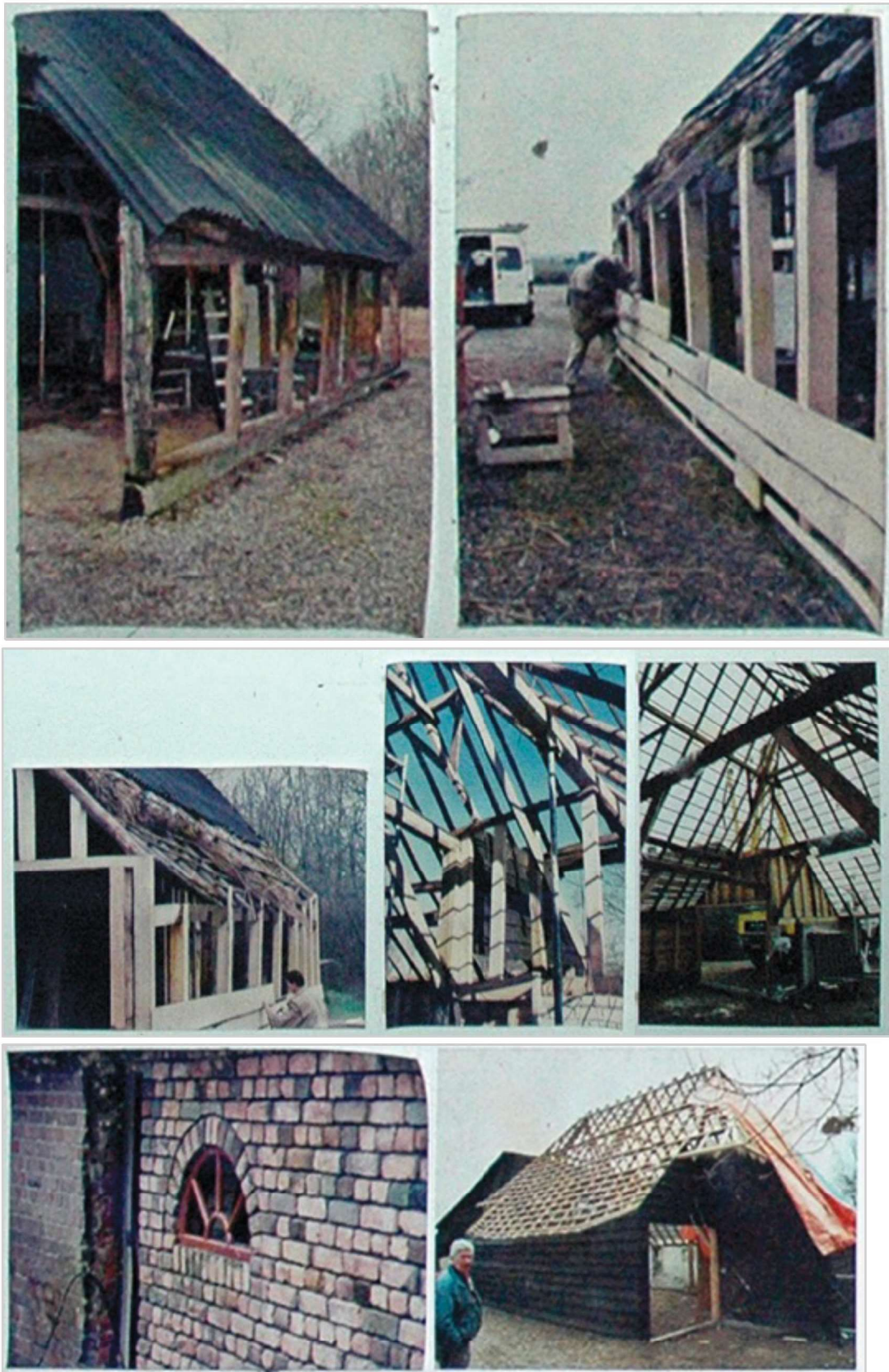
Afb. @ a t/m g: Zeven foto's uit een grotere verzameling waarmee men in @ de restauratie vastlegde. De foto's laten zien dat het, op de gebinten- en dakconstructie na, bijna volledige herbouw was. [Verzameling
