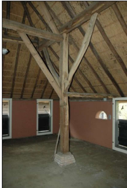
Afb. @ en @: Stijl van het eerste gebint links, zuidzijde ( o ) en noordzijde ( oo ).
