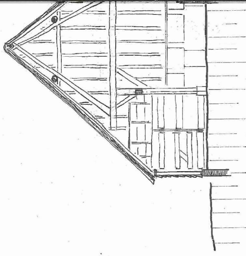
DOORSNEDE B-B
