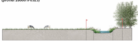
Huidig profiel Kleine Aa benedenloop (profiel 280001P0525)
