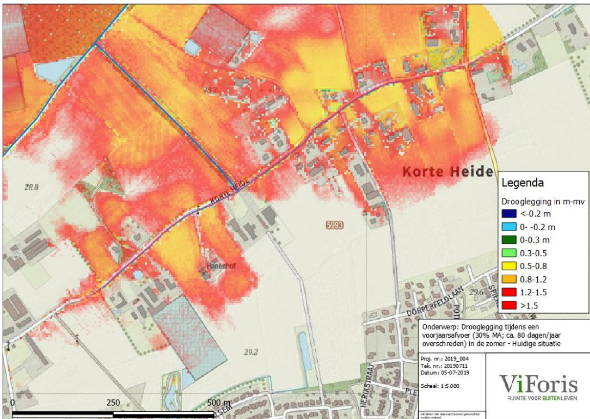
Figuur 5: Drooglegging tijdens een voorjaarsafvoer in de zomer (zomerweerstanden en zomerstuwstanden); ca. 80 dagen/jaar overschreden; in de huidige situatie op basis van de verbeterde modellering
