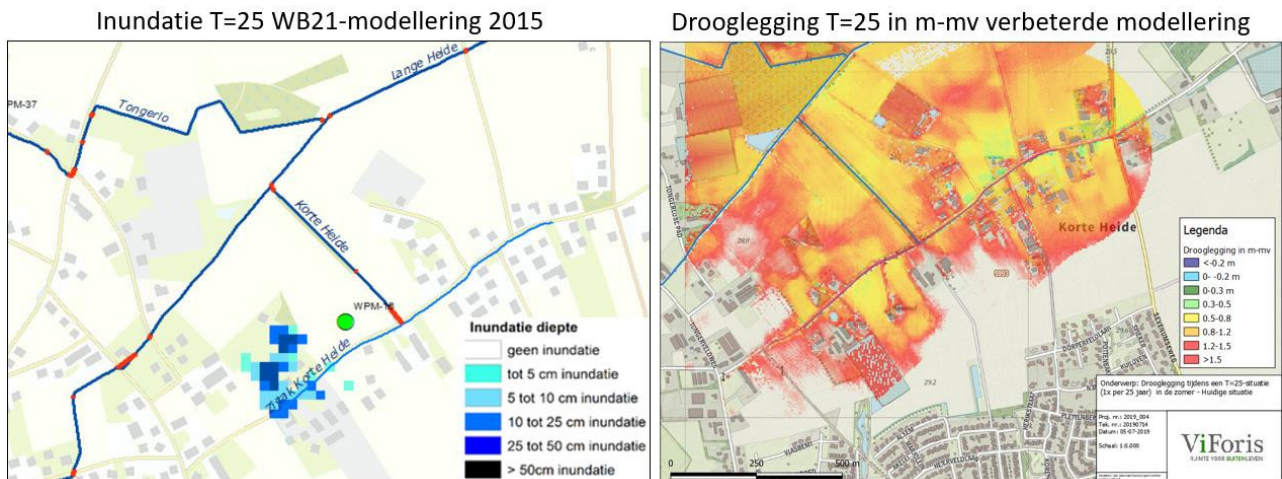
Figuur 8: Inundatie tijdens een T=25-situatie in de zomer op basis van de WB21-modellering van 2015 ten opzichte van de berekende drooglegging op basis van de verbeterde modellering (Q=2,0x MA; zomerstuwstanden met zomerweerstanden).
