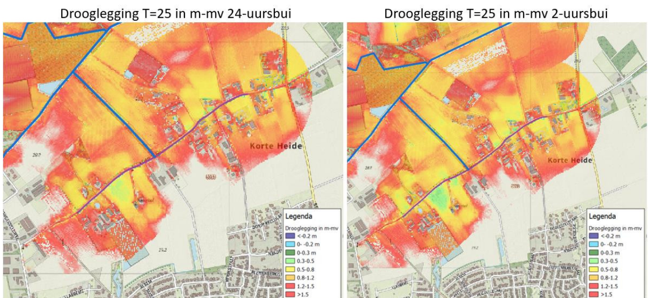
Figuur 9: Drooglegging tijdens een T=25 regenbui in 2 en 24 uur.
