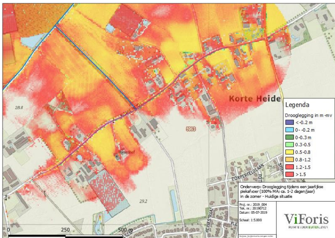
Figuur 6: Drooglegging tijdens een jaarlijkse piekafvoer in de zomer (zomerweerstanden en zomerstuwstanden); ca. 1-2 dagen/jaar overschreden; in de huidige situatie op basis van de verbeterde modellering
