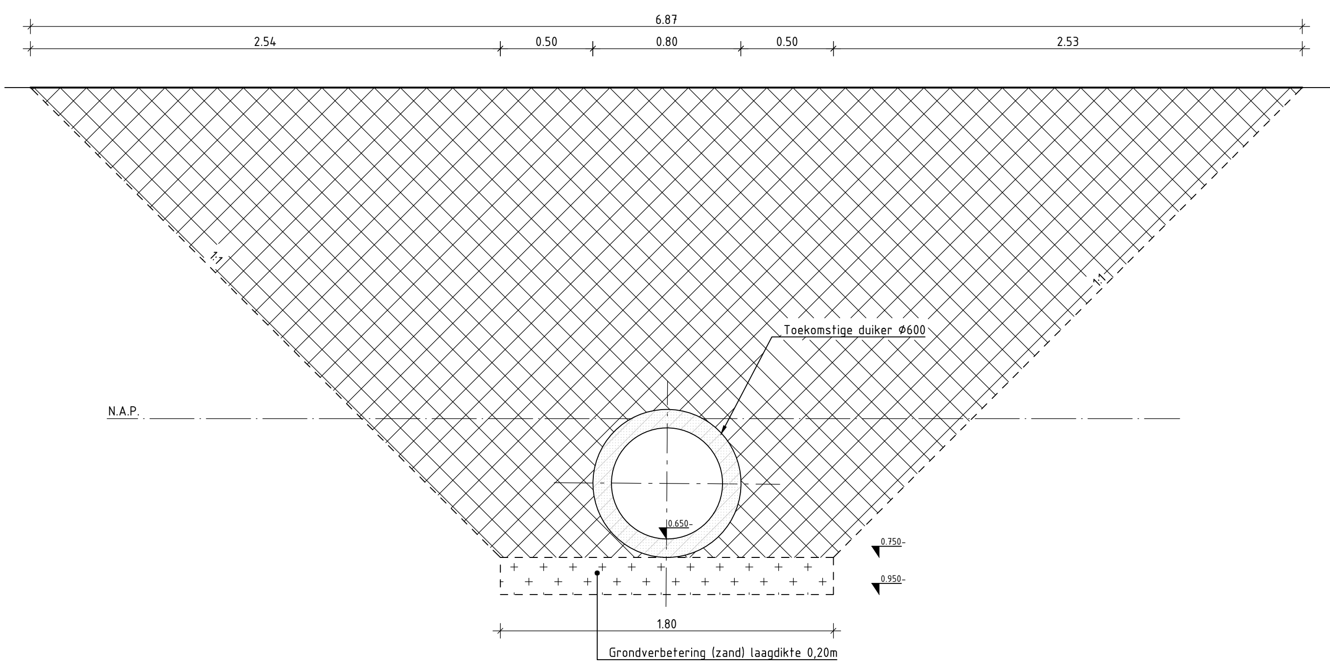
DOORSNEDE B-B (Toekomstige situatie) SCHAAL 1:20
