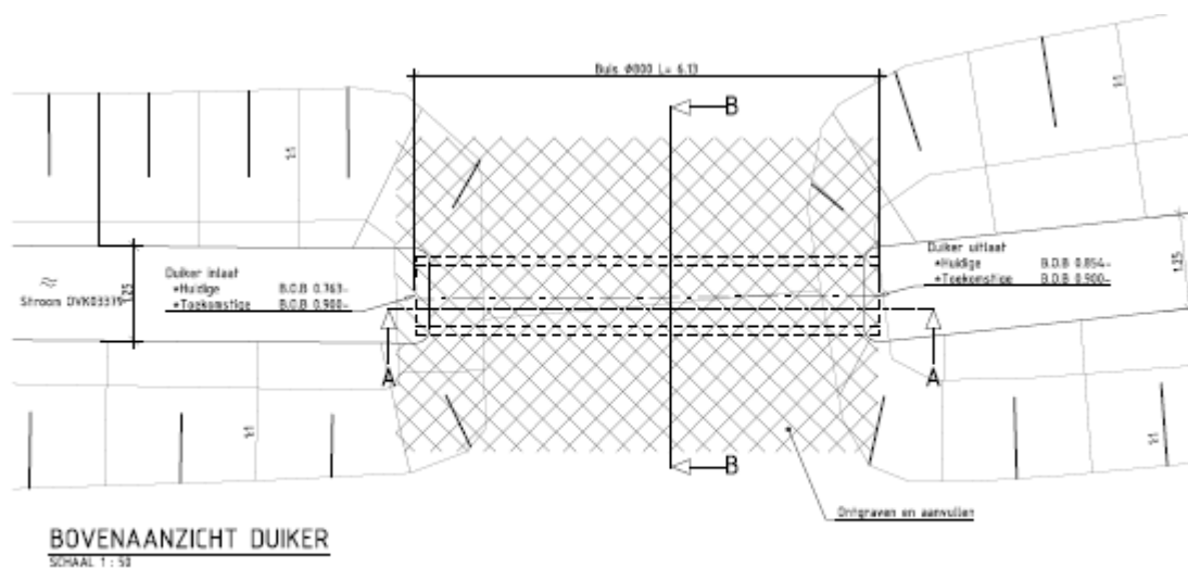
Figuur 10 Bovenaanzicht maatregel 3, bron: Lieveense
