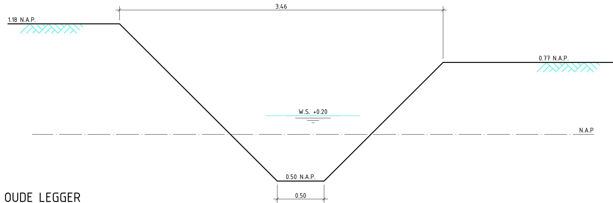
OUDE LEGGER SCHAAL 1:20
