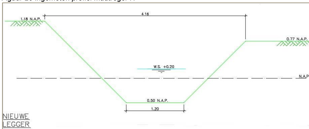
Figuur 21 Nieuwe legger profiel maatregel 7.
