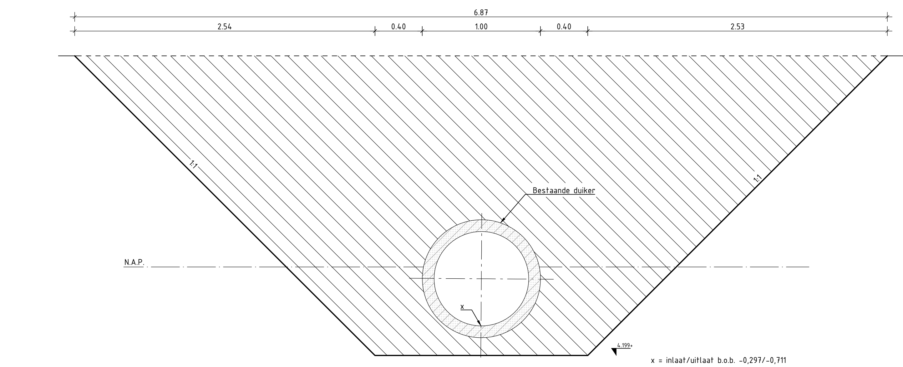
DOORSNEDE B-B (Bestaande situatie) SCHAAL 1:20
