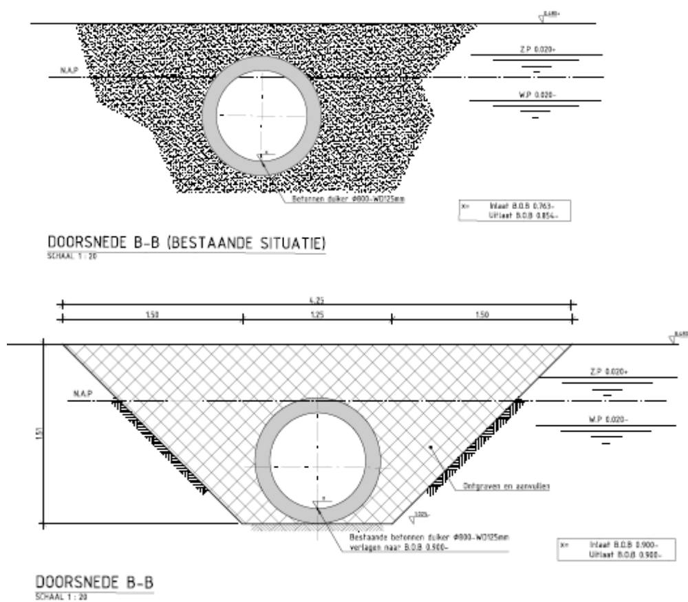
Figuur 11 Doorsnede maatregel 3 bestaand een nieuwe situatie, Bron: Lieveense
