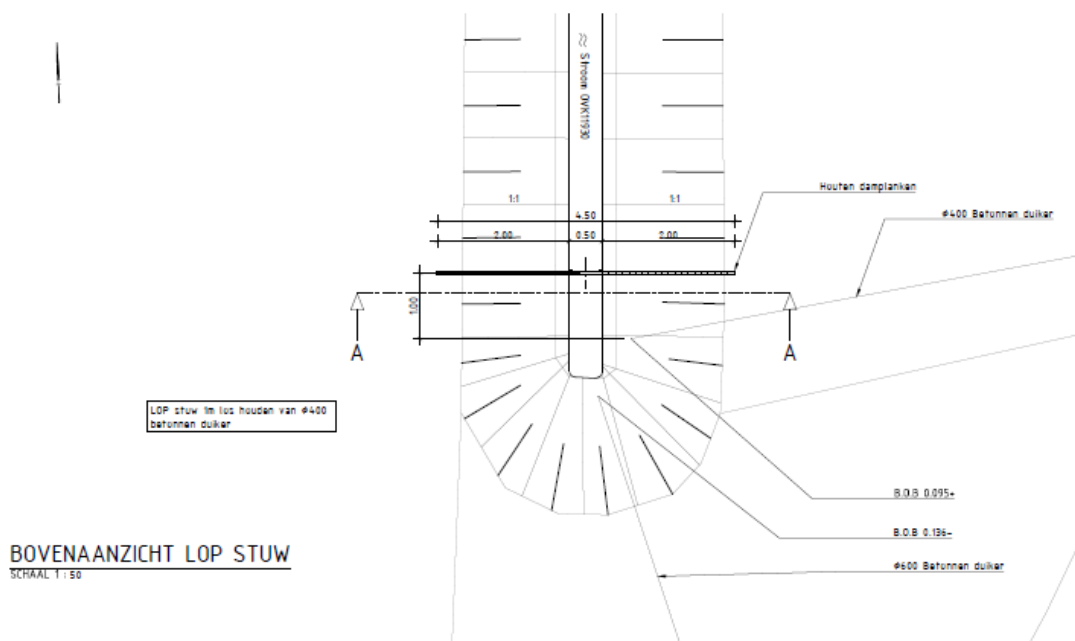
Figuur 16 Bovenaanzicht maatregel 5, bron: Lieveense
