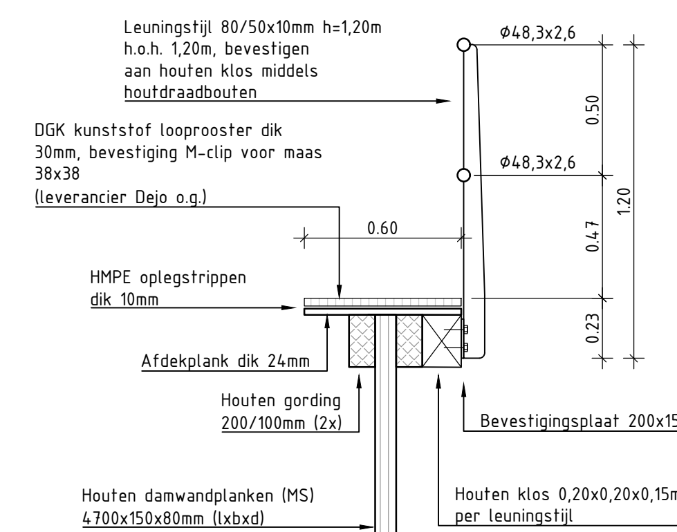
DOORSNEDE C SCHAAL 1:20
