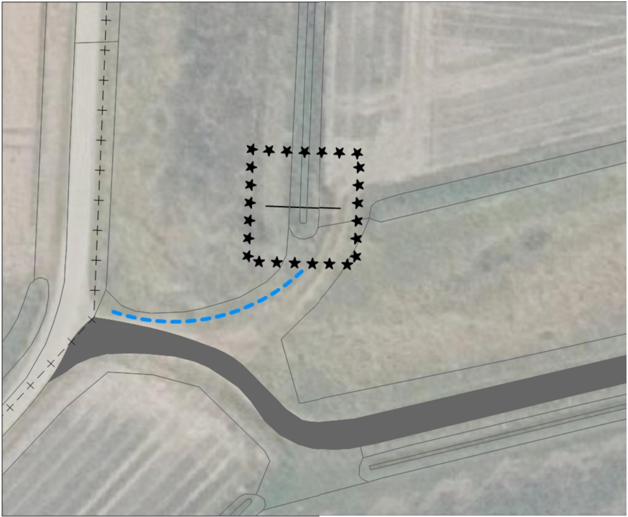
MAATREGEL 5: WERKGEBIED MET TIJDELIJKE BOUWWEG SCHAAL 1 : 500
