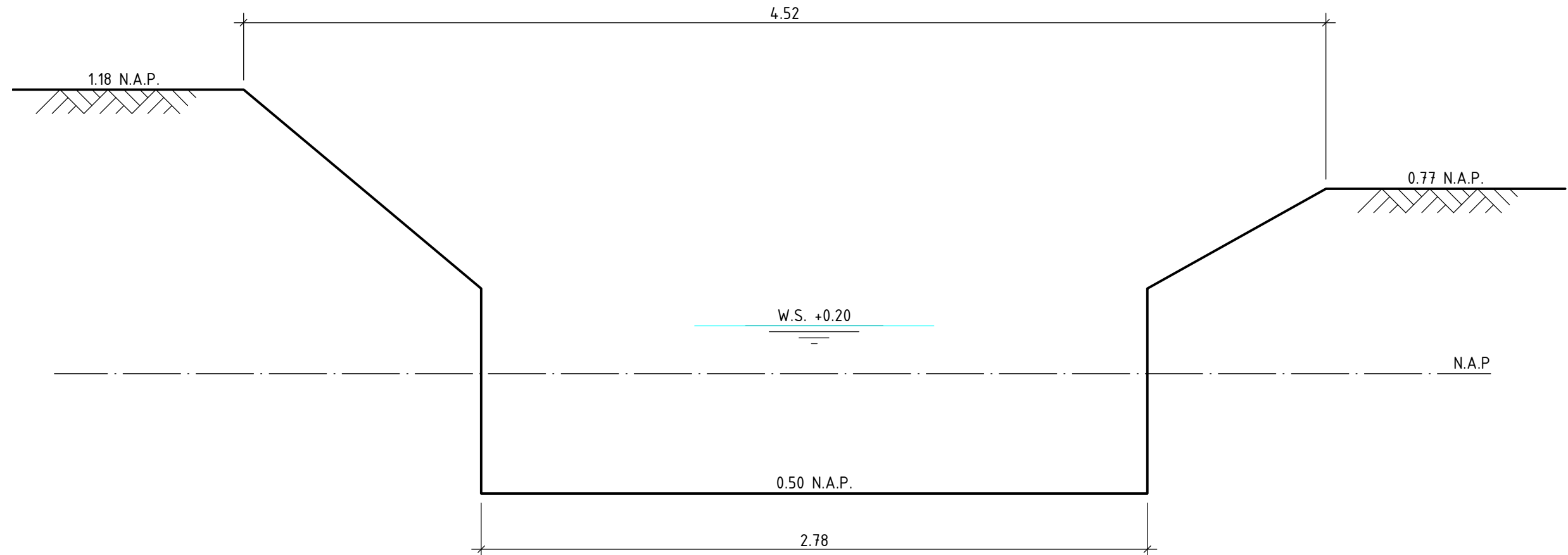
INGEMETEN PROFIEL SCHAAL 1:20
