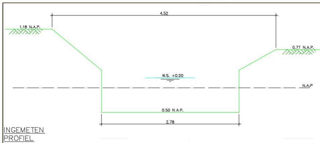
Figuur 20 Ingemeten profiel maatregel 7.
