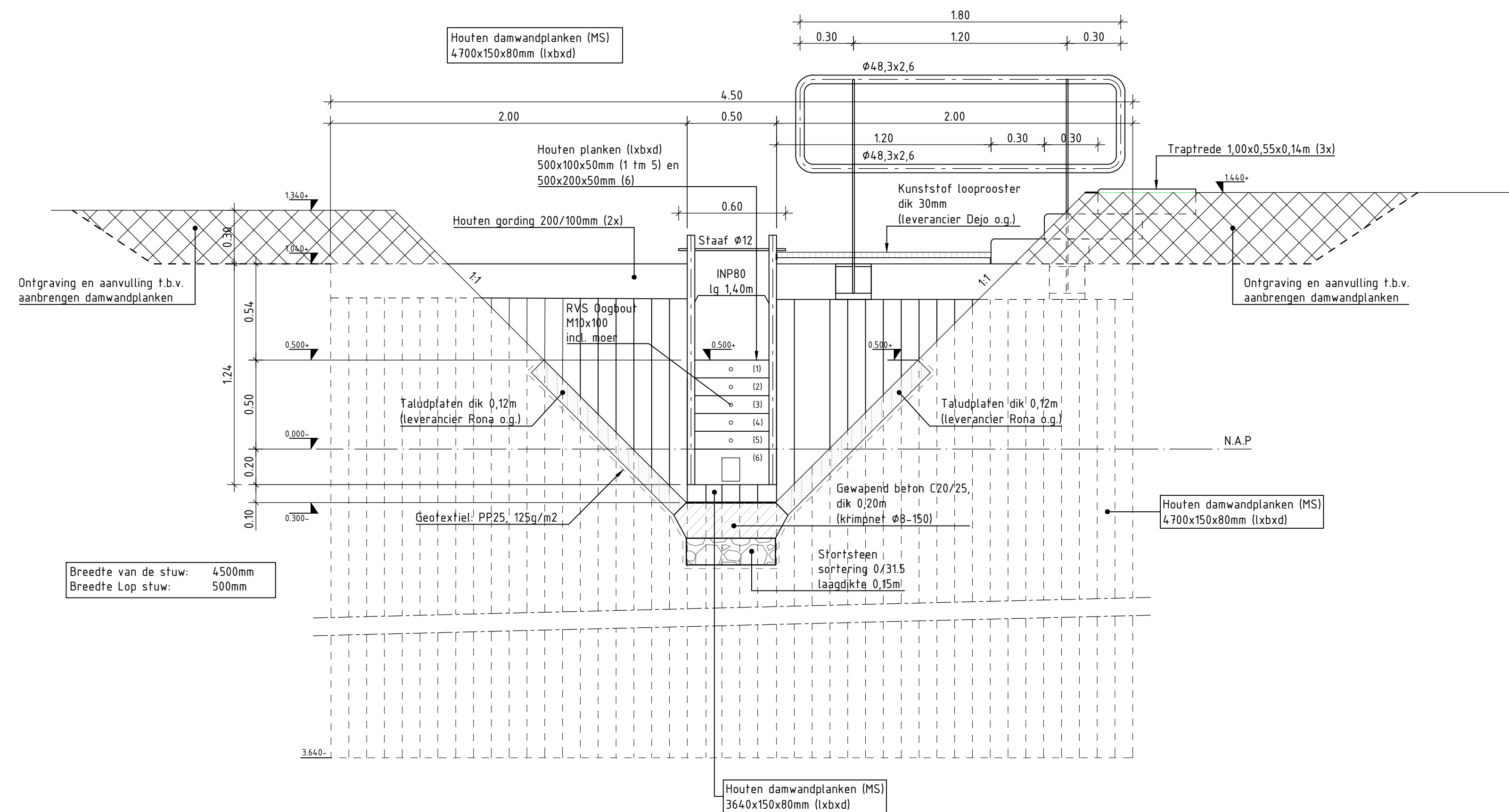
DOORSNEDE A-A SCHAAL 1:20
