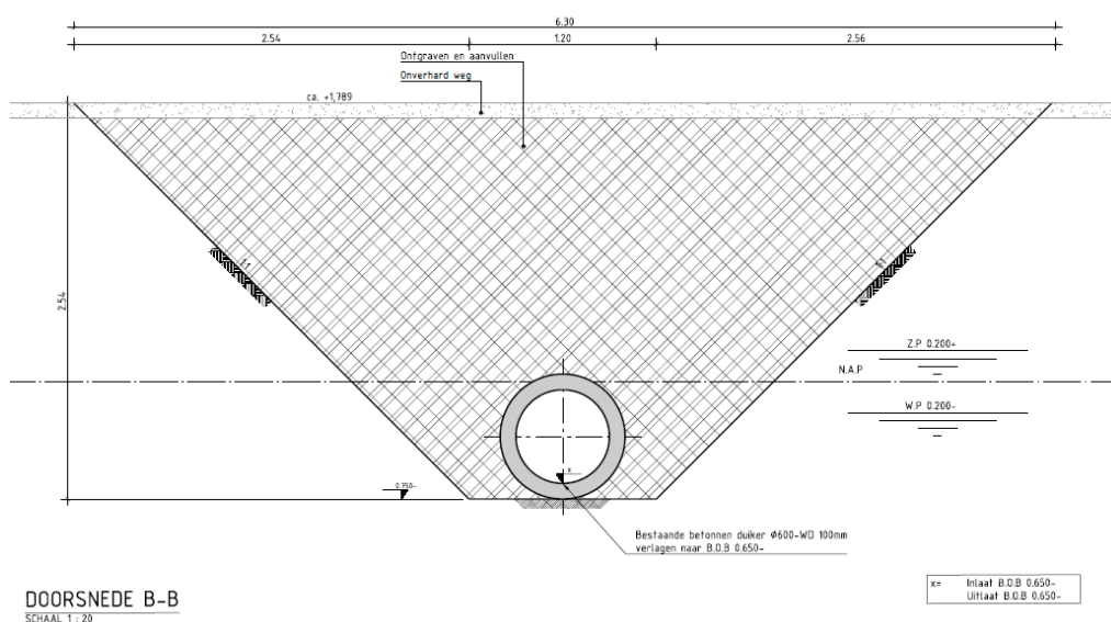
Figuur 19 Vooraanzicht maatregel 6, bron: Lieveense
