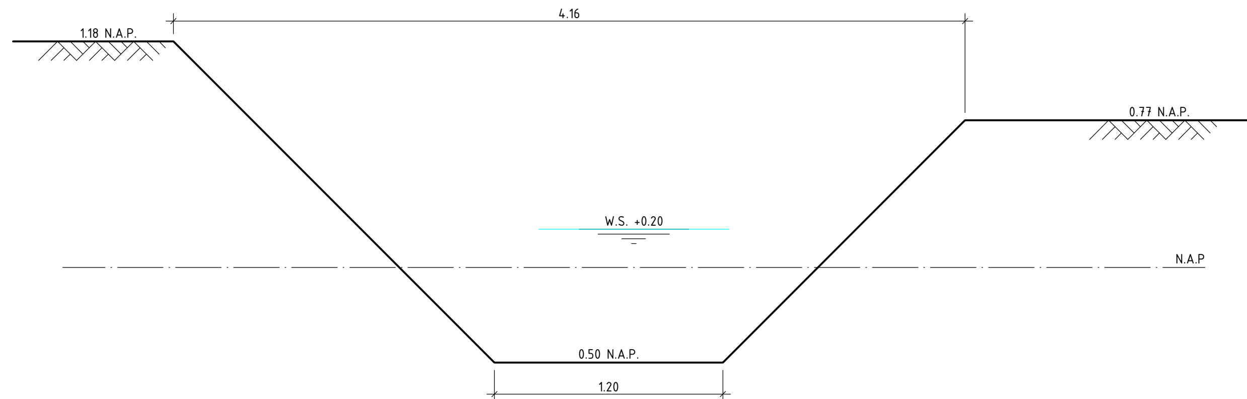
NIEUWE LEGGER SCHAAL 1:20
