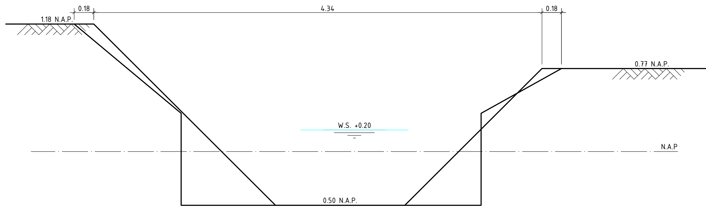
NIEUWE LEGGER + INGEMETEN PROFIEL SCHAAL 1:20
