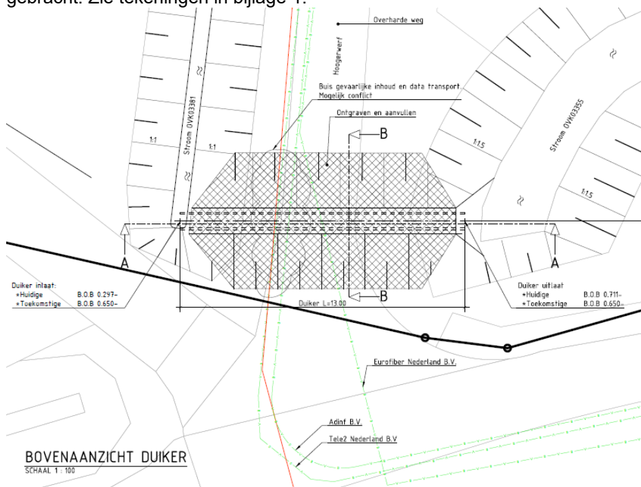
Figuur 18 Bovenaanzicht maatregel 6, bron: Lieveense
