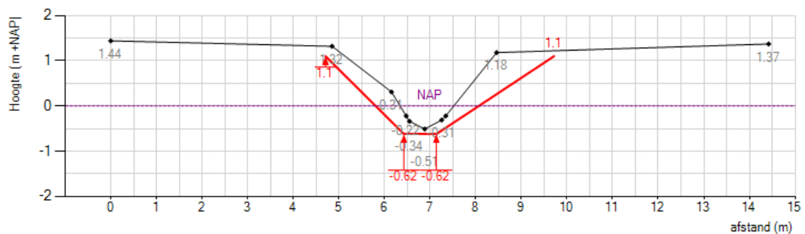
Figuur 3: Ingrep 6. Dwarsdoorsnede PRO15523 (10/28/2013) met de (huidige) vaste bodem (zwarte lijn) en het leggerprofiel (rode lijn), Bron: Waterschap Brabantse Delta.
