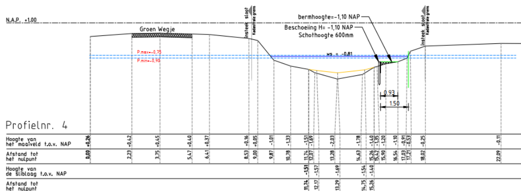
Fig. 2 Principeschets aanleg natuurvriendelijke oever langs het Groenewegje
