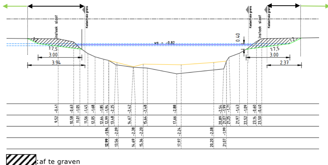
Fig. 1 Principeschets aanleg natuurvriendelijke oever
