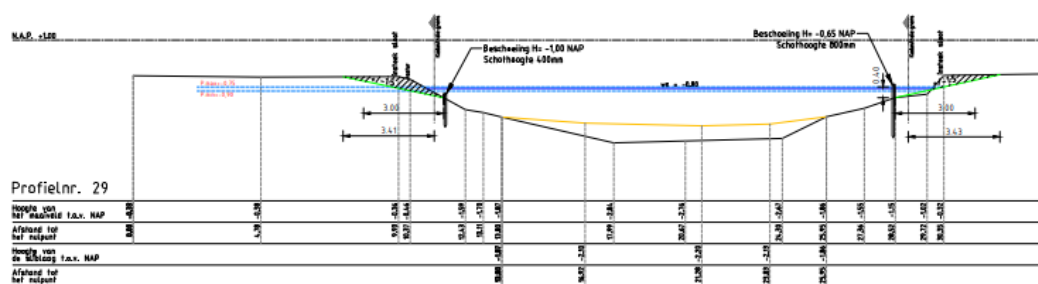
Fig. 3 Principeschets aanleg natuurvriendelijke oever ten noorden van het Nekkeveld
