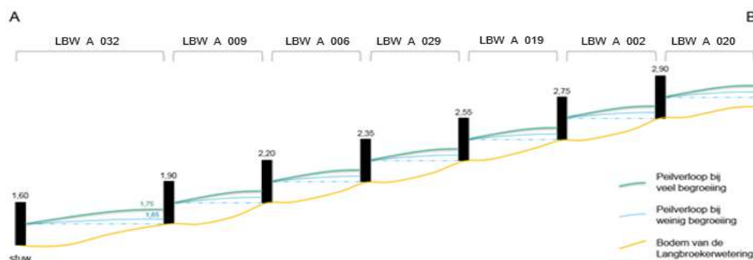
Dwarsdoorsnede van de Langbroekerwetering. Bij de stuwen worden de peilen genoemd waarop die stuw is ingesteld. Daarnaast wordt het peilverloop in de watergang getoond.
