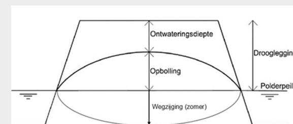
Schematische weergave van de ontwatering en drooglegging
