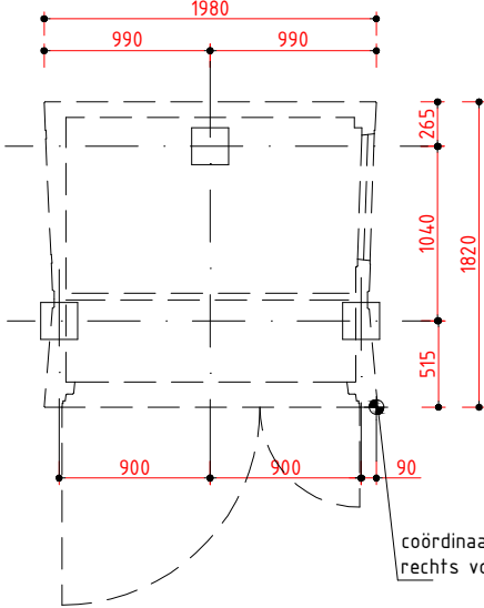
PALENPLAN
