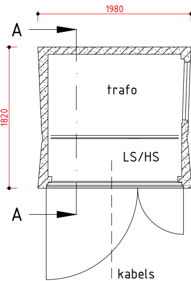
PLATTEGROND
