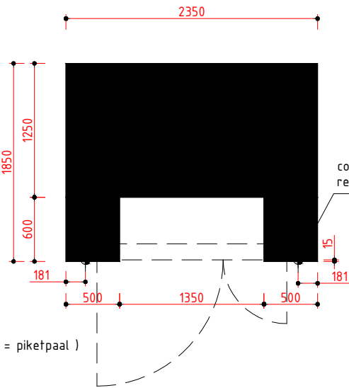
FUNDERING GESTABILISEERD ZAND dikte volgens opgave constructeur
