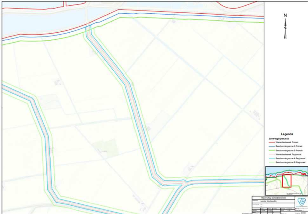
waterkeringszone Emelissedijk
