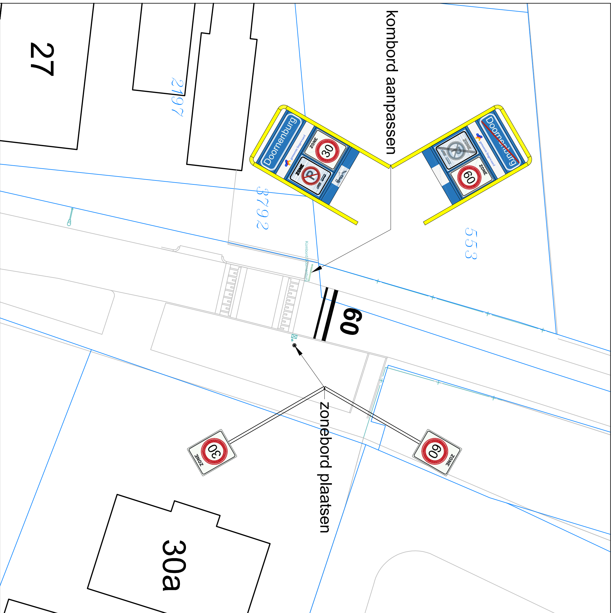
2. Poortconstructie Rijnstraat nabij woning no. 30A
