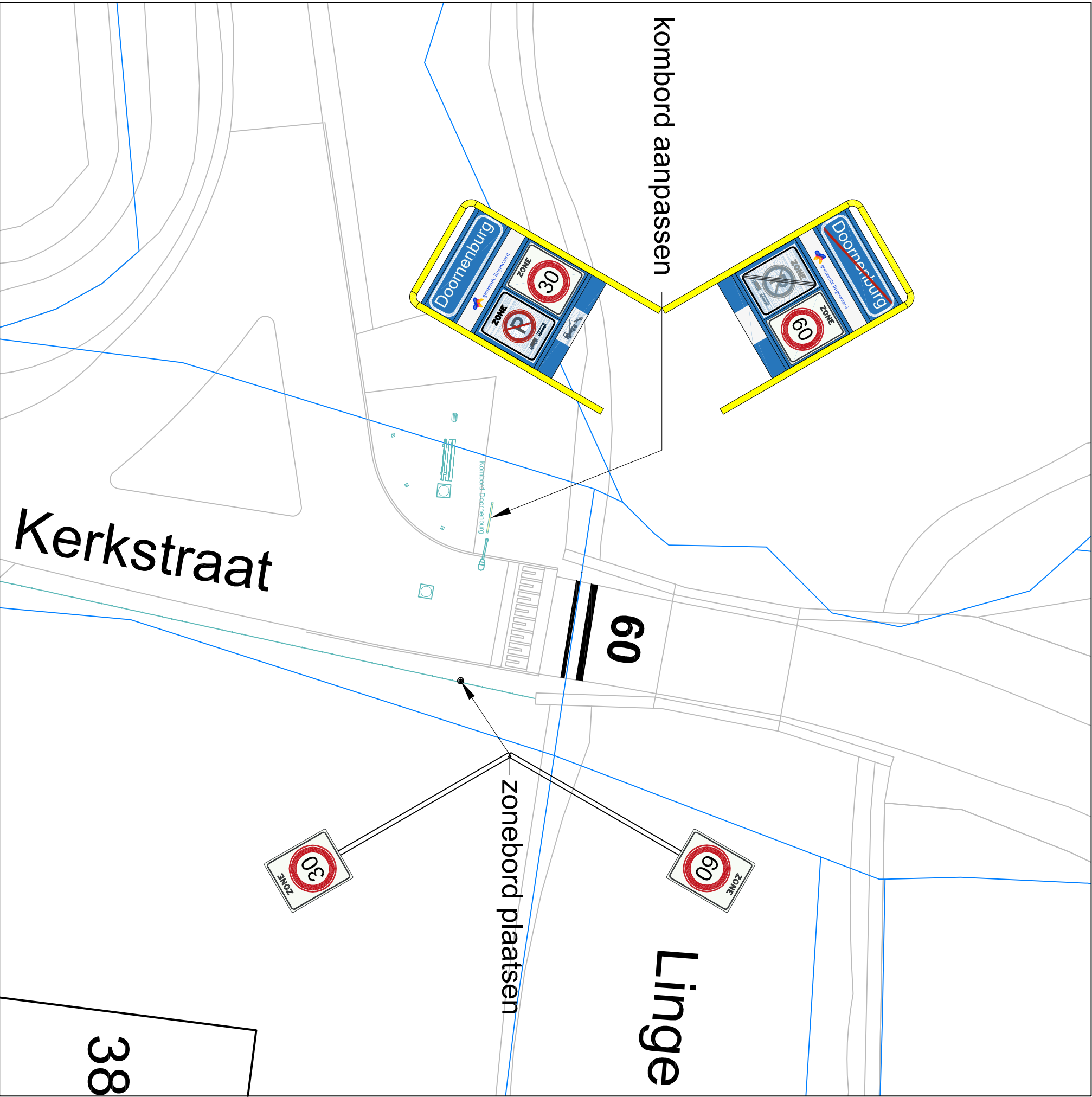
1. Poortconstructie Kerkstraat nabij Linge
