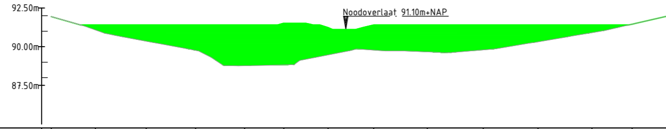
Dwarsprofiel DP-02 Schaal 1:500
