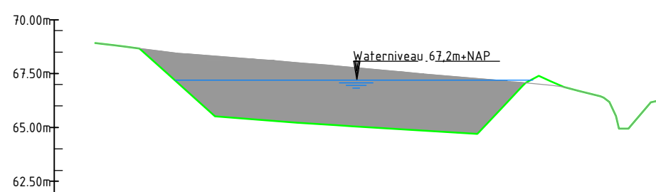
Dwarsprofiel DP-04 Schaal 1:500
