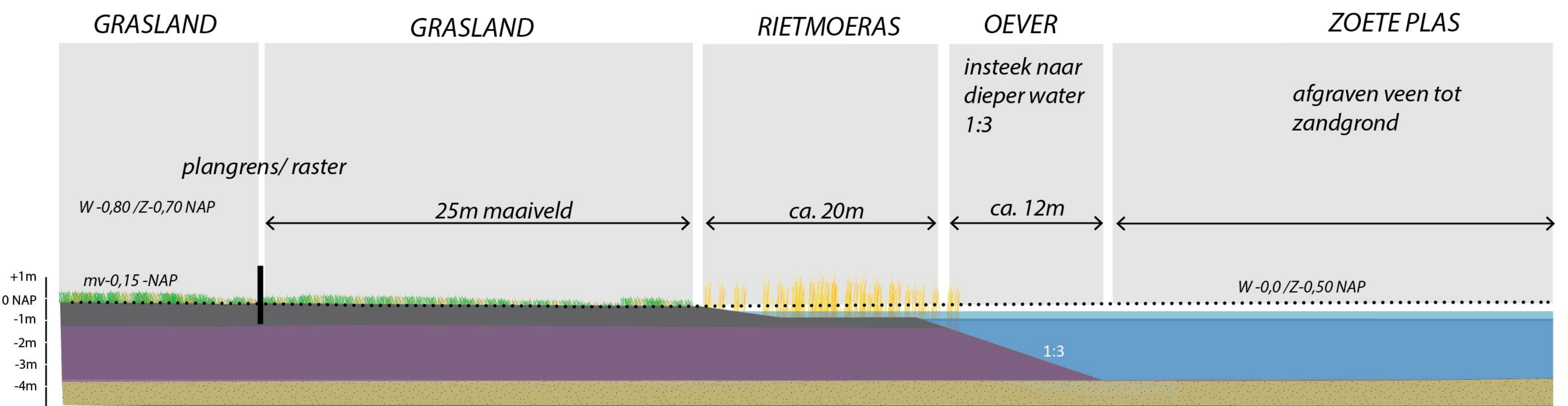
Profiel E overgang landbouw - zoete plas
