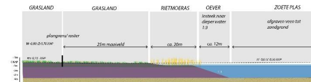
Profiel E overgang landbouw - zoete plas
