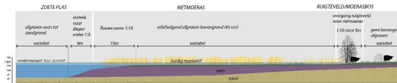
Profiel A overgang ruigte - rietmoeras - zoete plas
