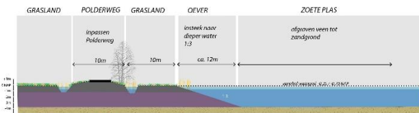
Profiel D overgang Polderweg - zoete plas
