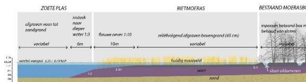
Profiel B overgang bestaand bos - rietmoeras - zoete plas
