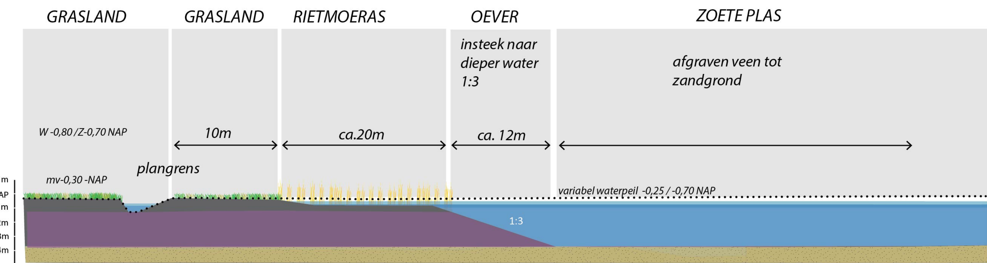
Profiel F overgang landbouw - zoete plas
