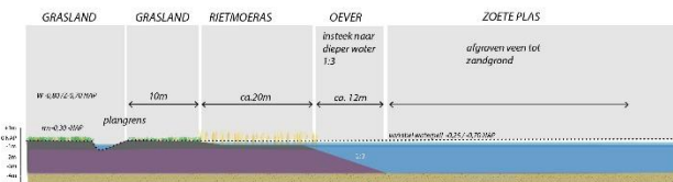
Profiel F overgang landbouw - zoete plas
