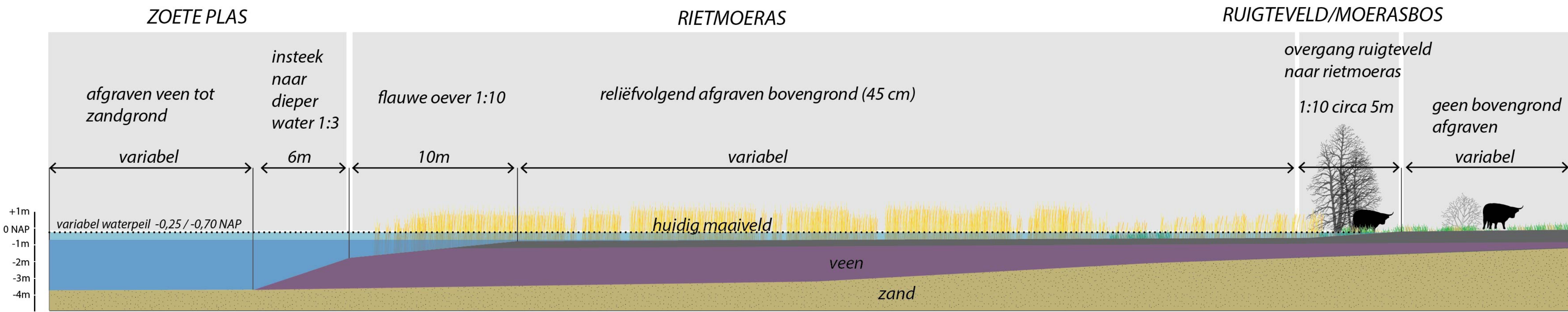
Profiel A overgang ruigte - rietmoeras - zoete plas
