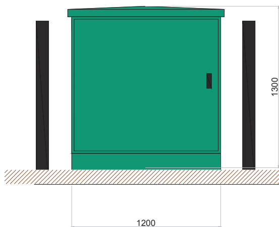
Voor aanzicht
