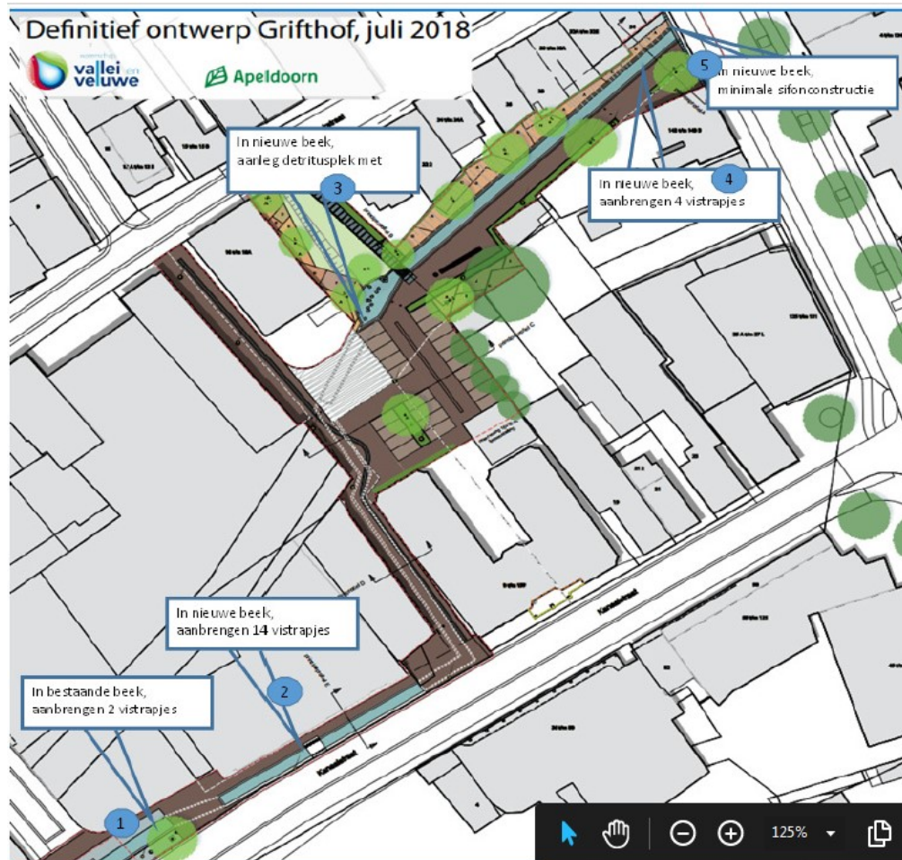
Figuur 5 Maatregelen beekprik
