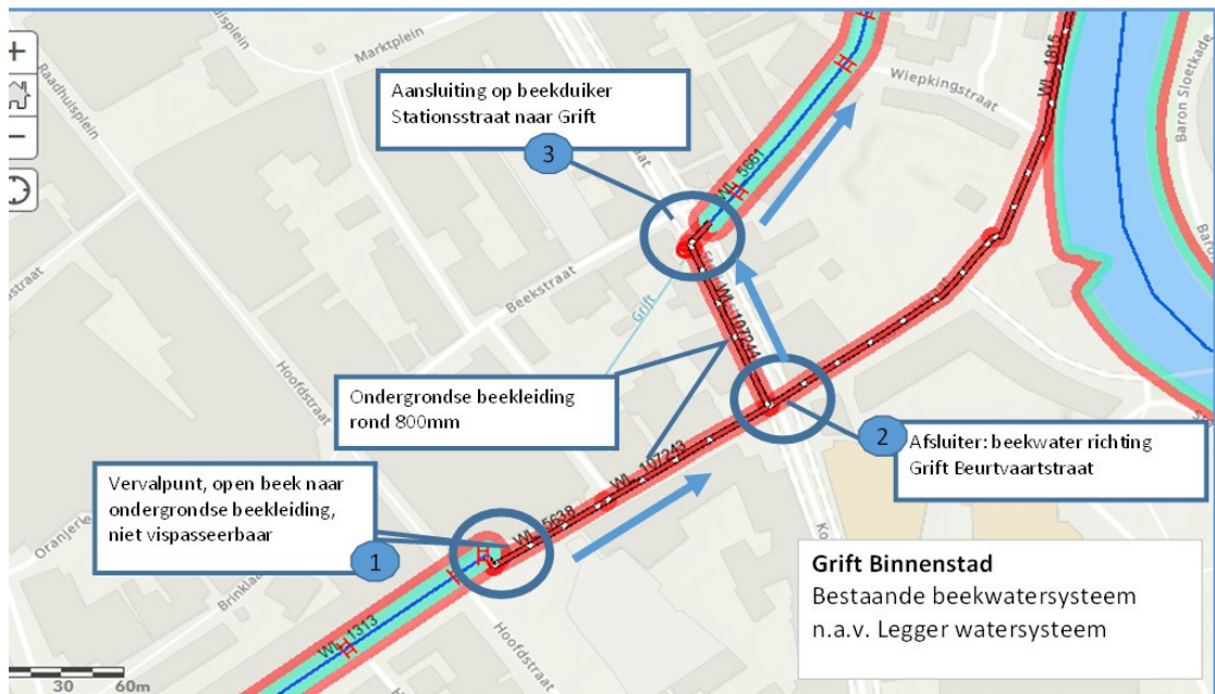
Figuur 2 Bestaand beekwatersysteem
