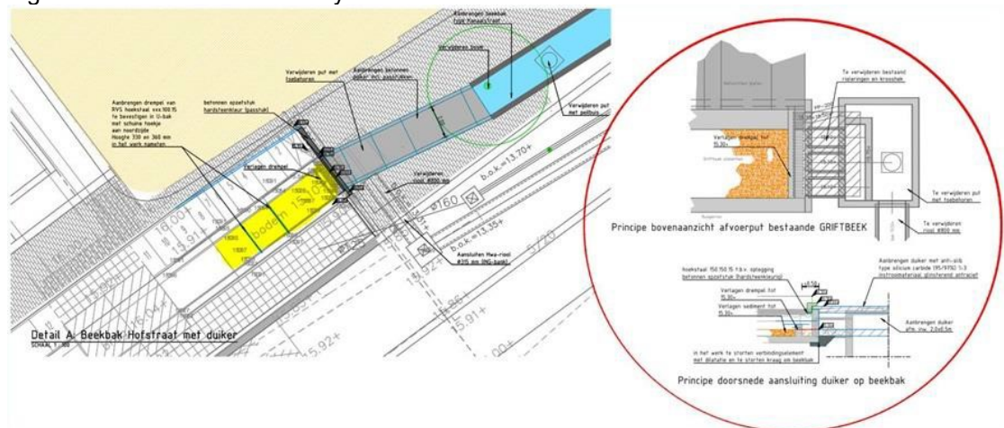
Figuur 3 Vervalpunt Kanaalstraat: open beek gaat over in een ondergrondse beekleiding, rond, 800 mm doorsnede, via een groot vervalpunt. Stroomopwaarts niet vispasseerbaar.
