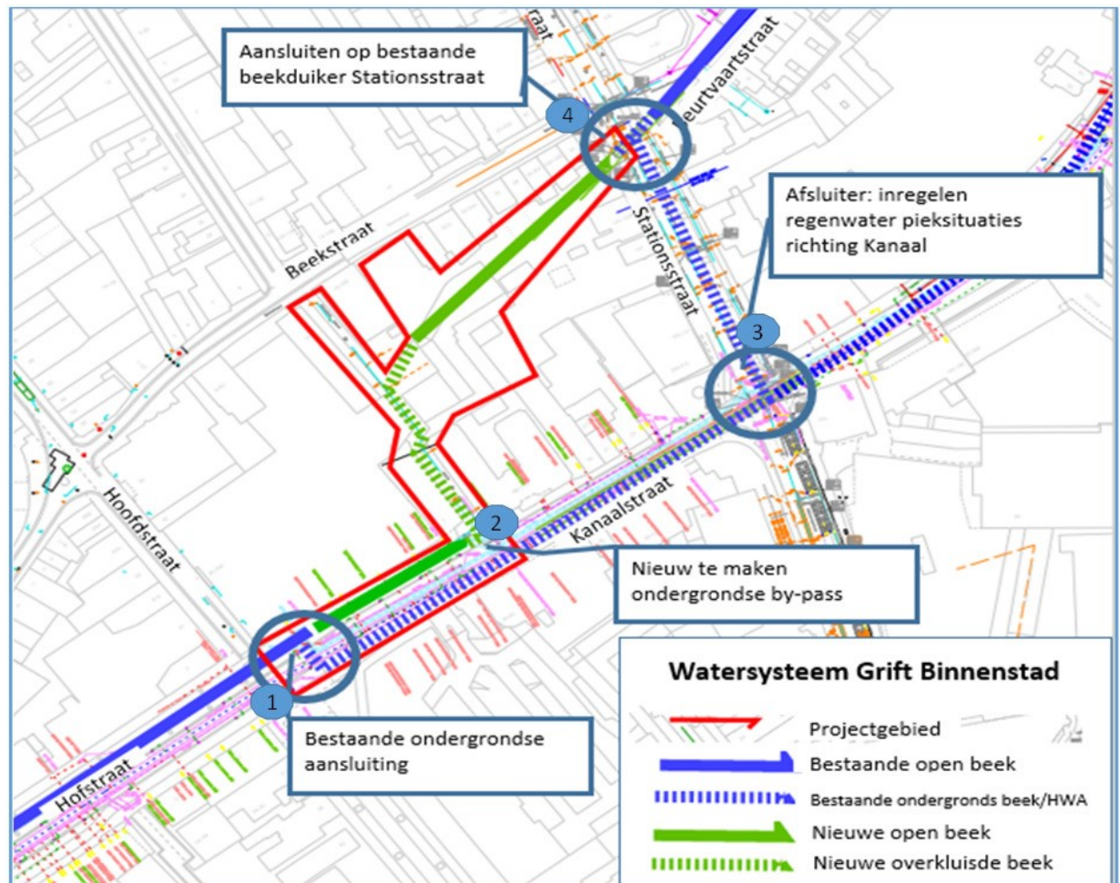
Figuur 4. Nieuwe situatie, met vispasseerbaar ondergronds deel
