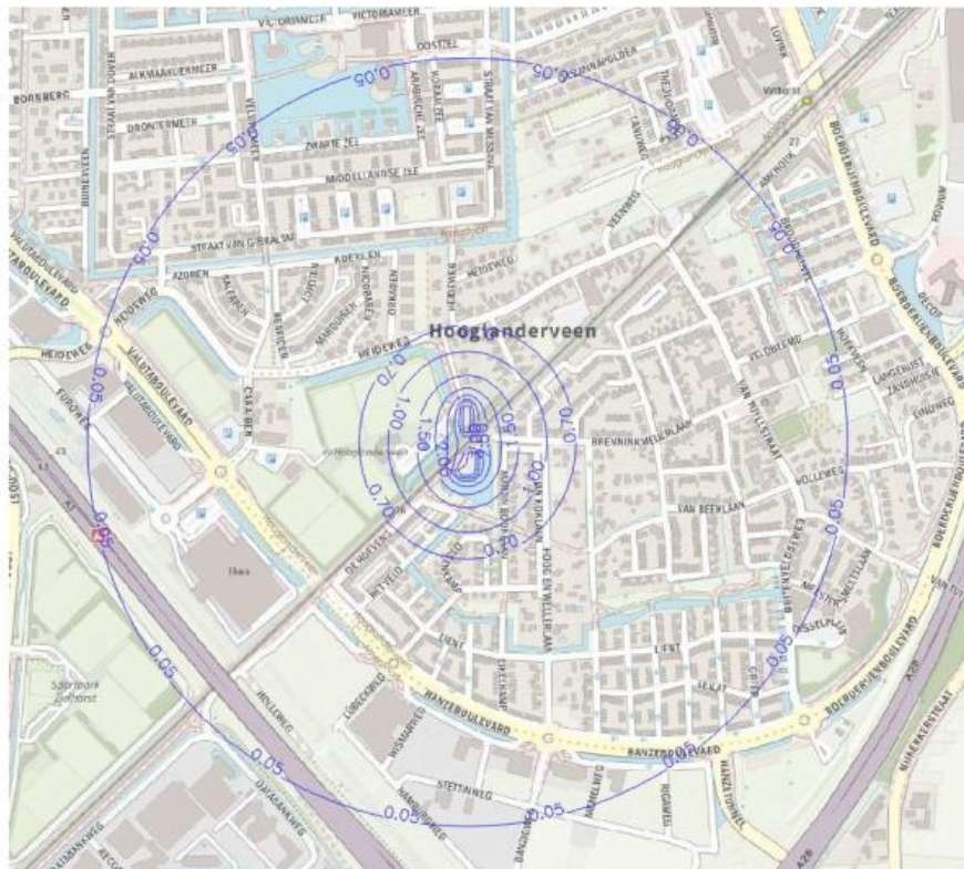
Verlaging in meter t.o.v. GHG in laag 3
