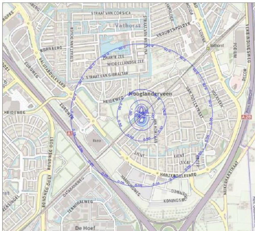
Figuur 5.3.2 Verlaging in meter t.o.v. GLG in laag 3
