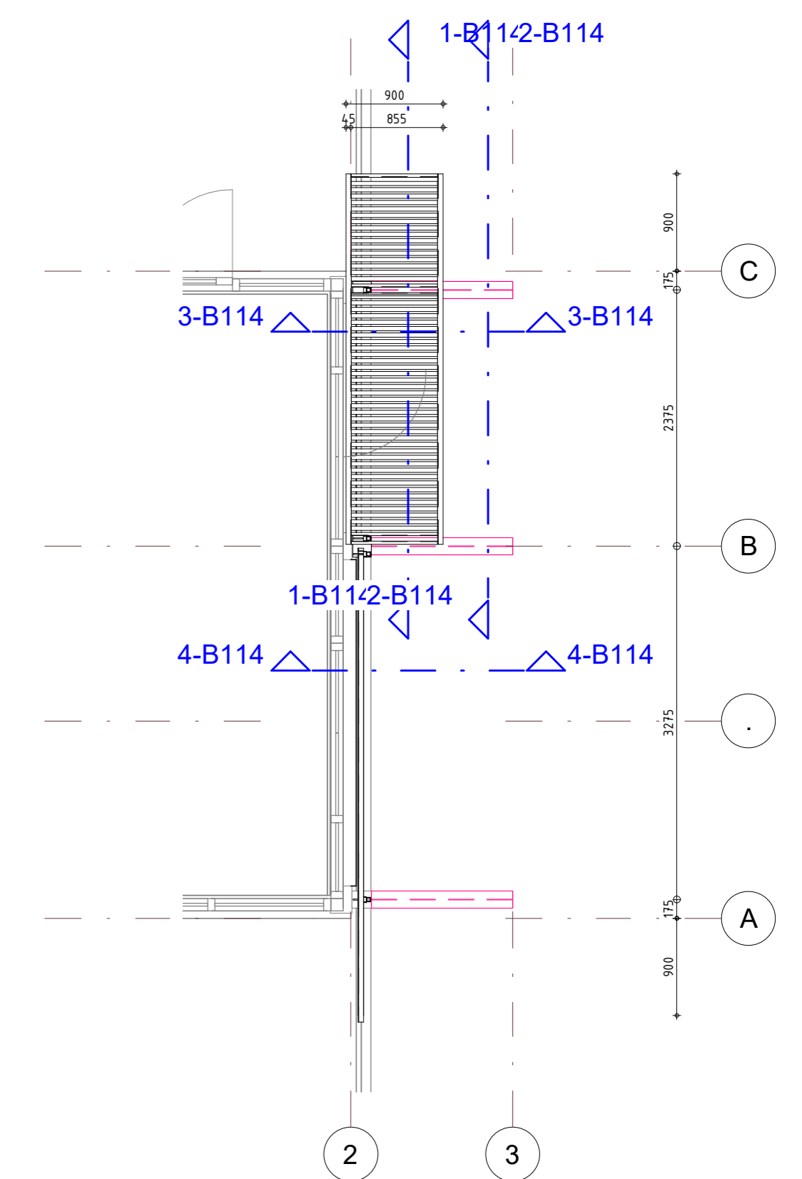
Plattegrond (1:50)
