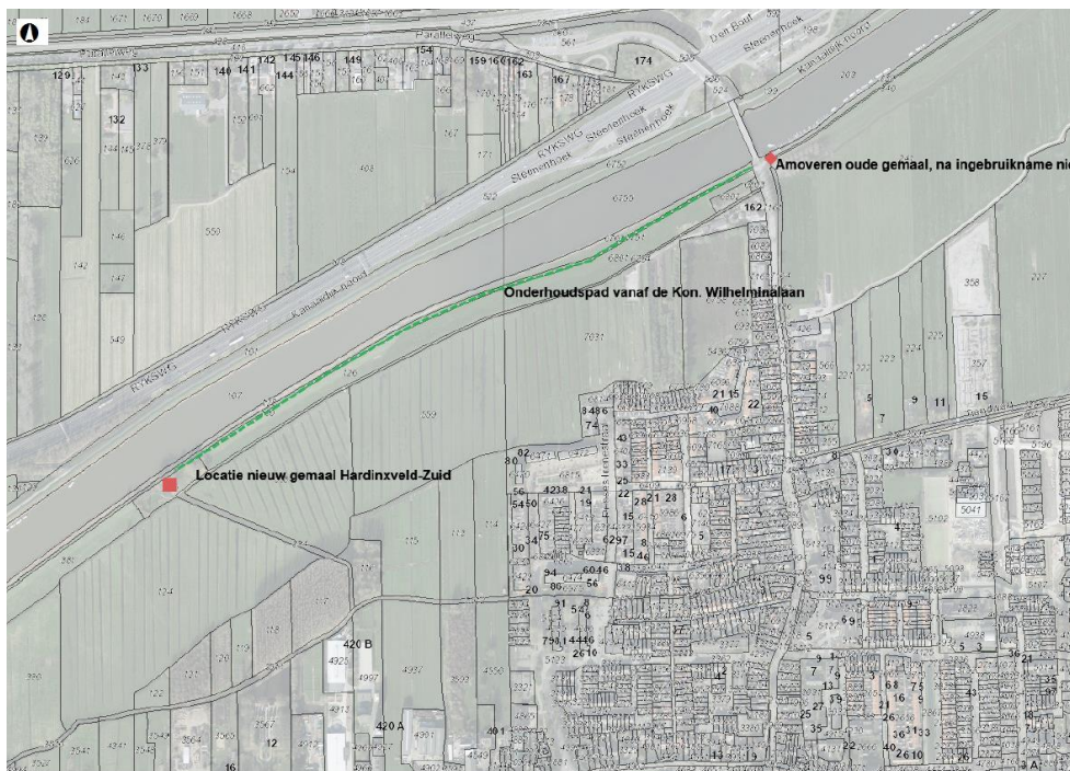
Figuur 1: locatie nieuw en bestaand gemaal Hardinxveld Zuid te Hardinxveld-Giessendam
