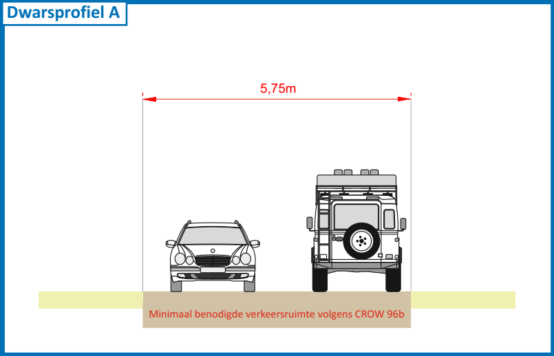
Dwarsprofiel A
