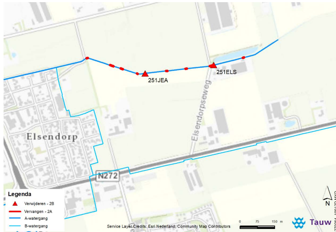
Figuur 3.2 Locatie geplande vervanging duikers
