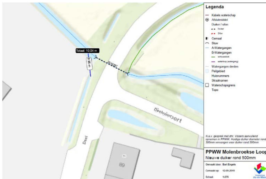
Figuur 2.4 Locatie te vervangen dijk langs Deel
