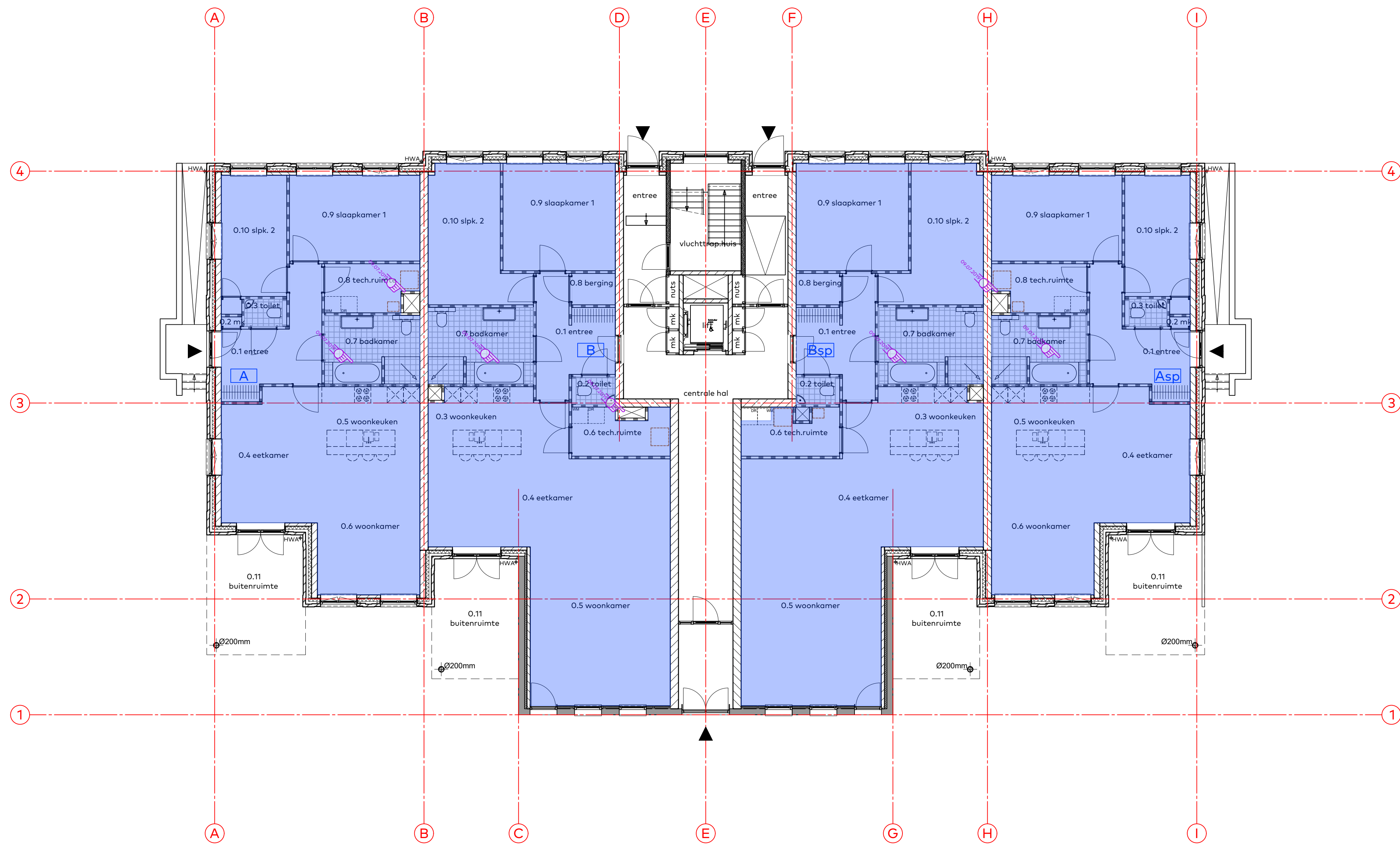
Begane grond GO appartement A = 102,3 m 2 GO appartement B = 135,8 m 2
