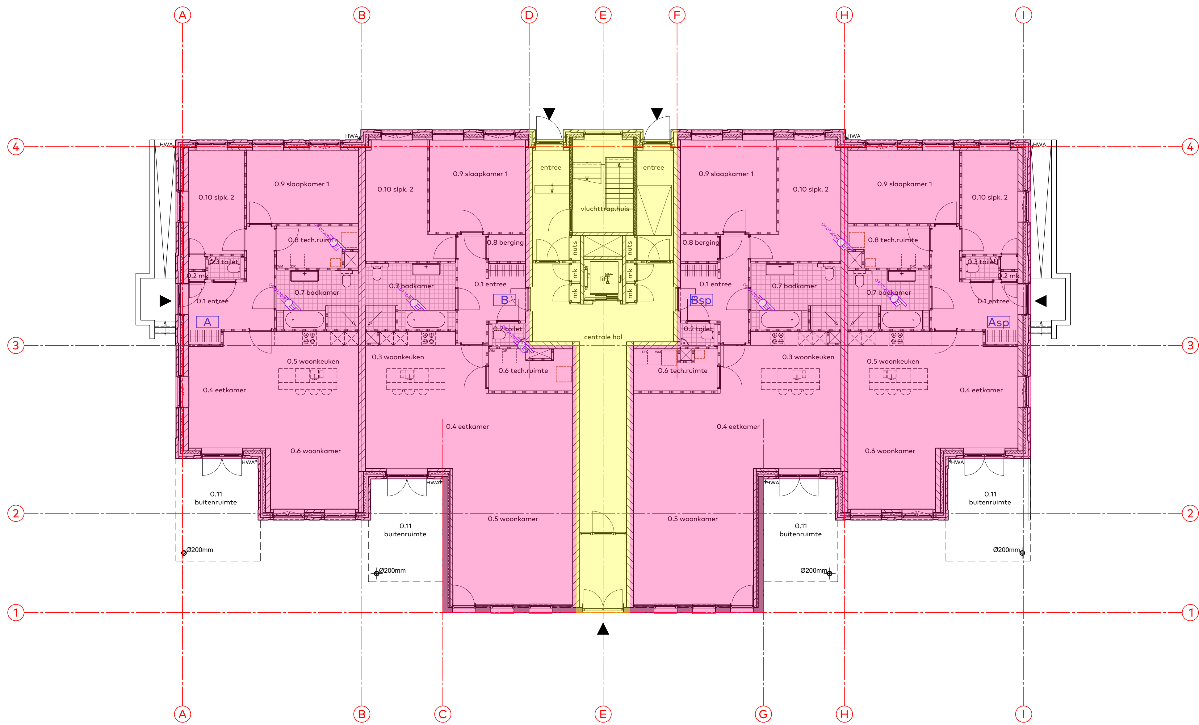
Begane grond BVO appartement A = 120,5 m 2 BVO appartement B = 152,2 m 2
