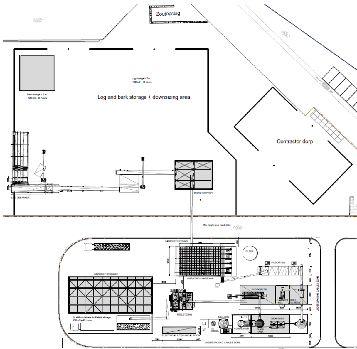
Figuur 6: Schets van locatie en indeling demoplant
