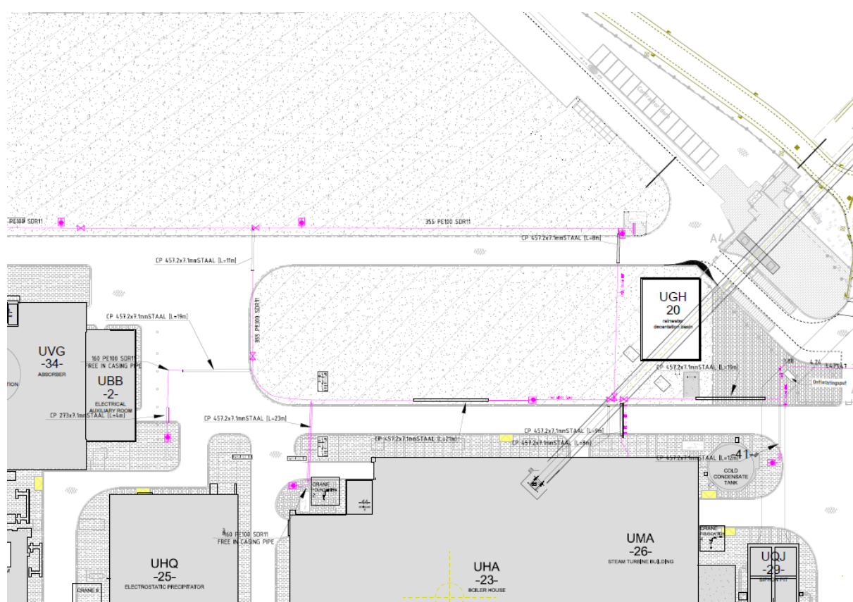
Figuur 8: Blusvoorzieningen rondom de geplande locatie van de demoplant. Roze stippen zijn de kranen. (bron: PPR)
