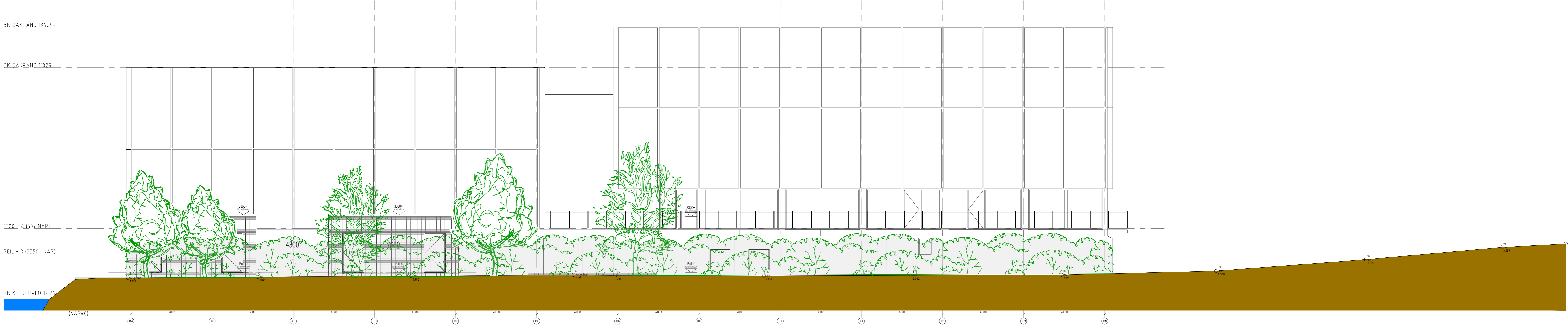
Oostgevel - Nieuwe situatie Schaal 1:100
