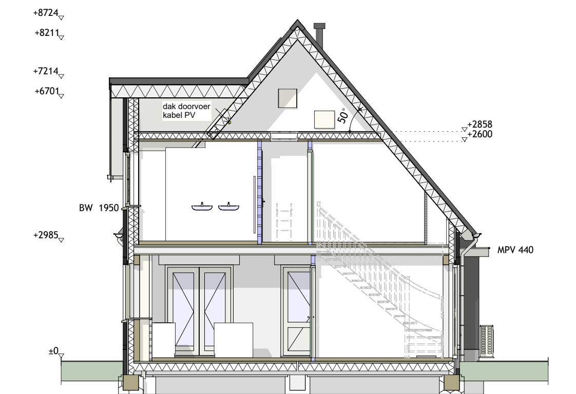
Doorsnede hoofdbouw
