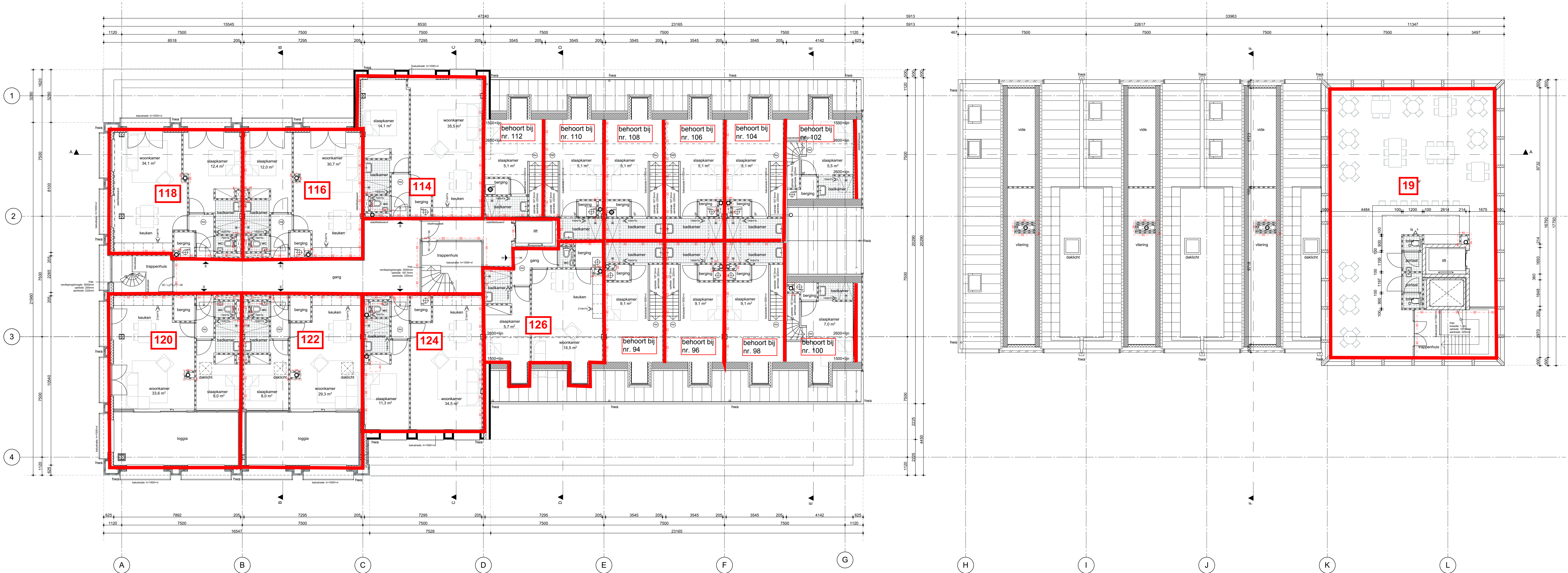
4e verdieping peil = +1250m
