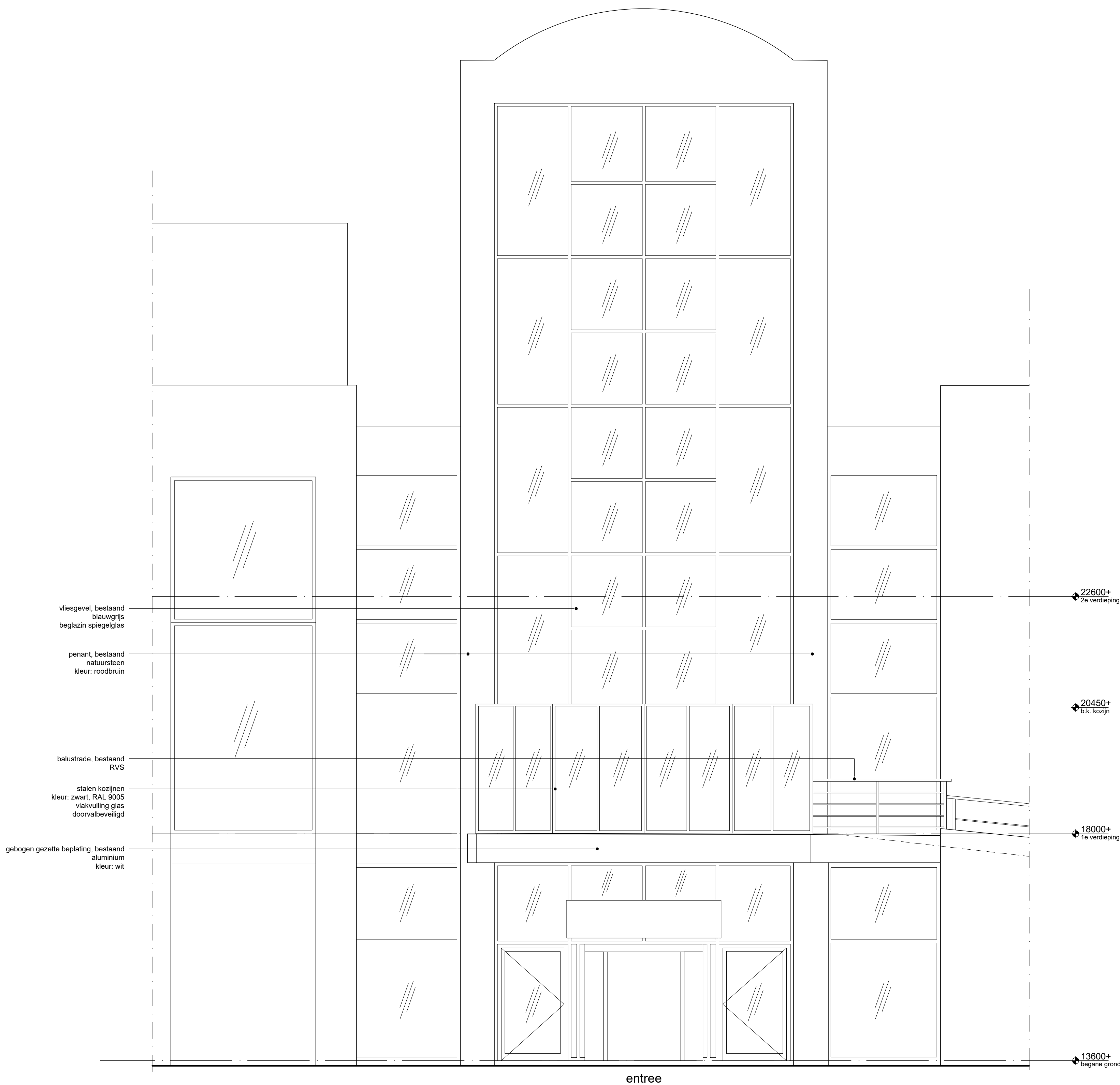
1 aanzicht waalkade - nieuw 1:50
