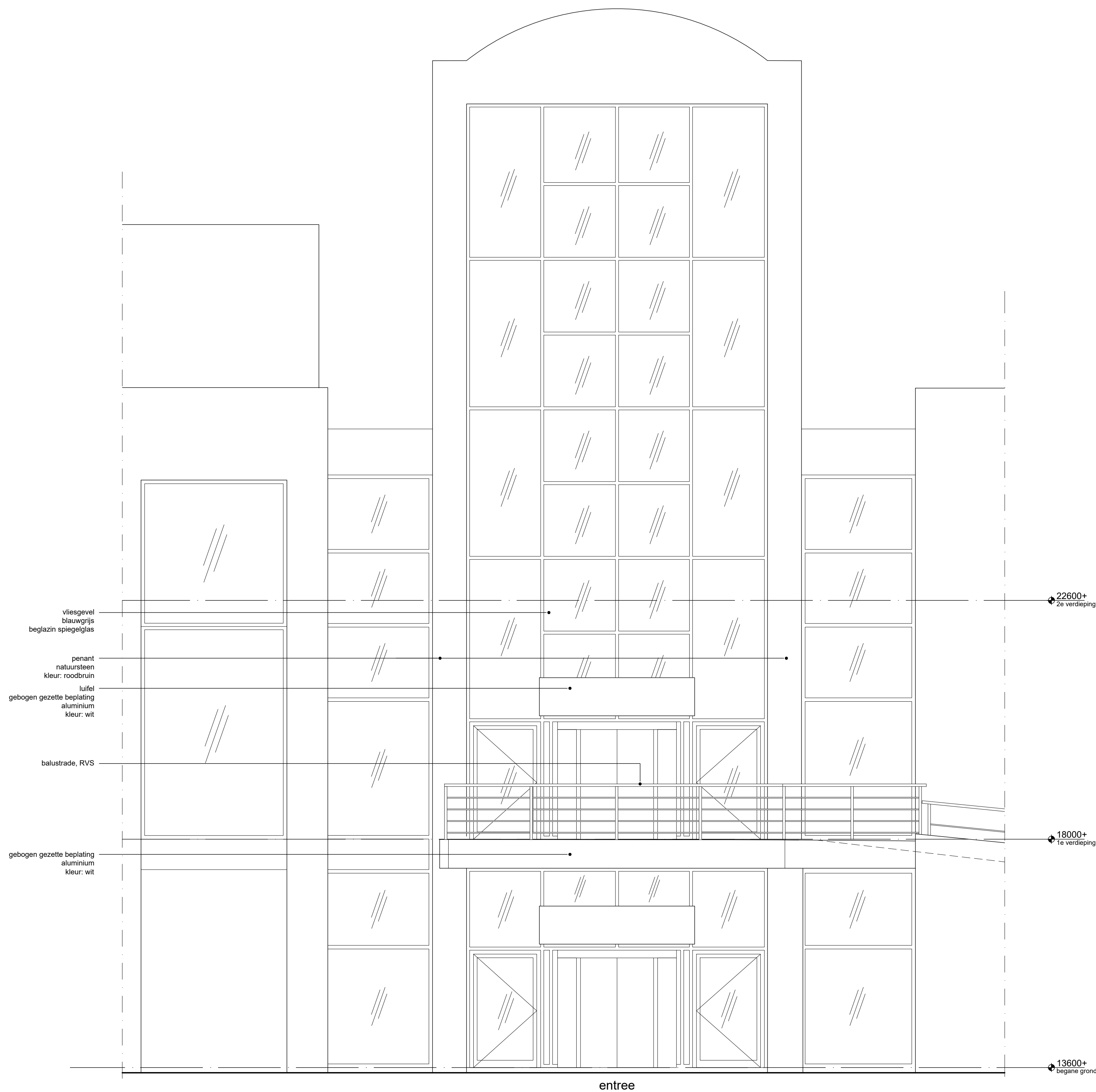
1 aanzicht waalkade - bestand 1:50
