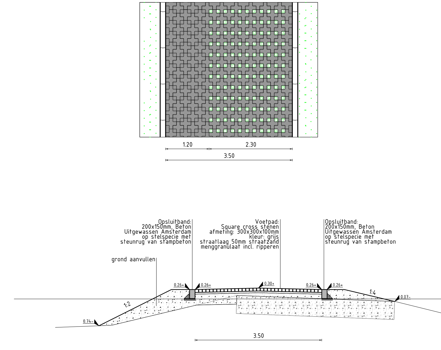
DOORSNEDE D SCHAAL 1 : 50
