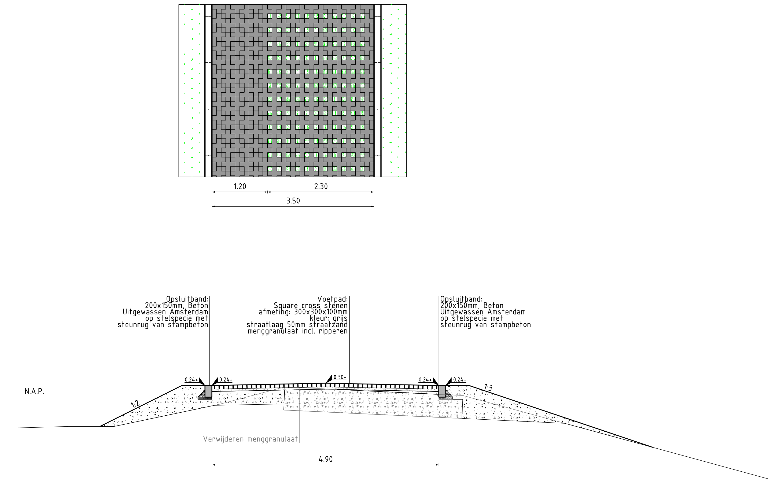
DOORSNEDE C SCHAAL 1 : 50
