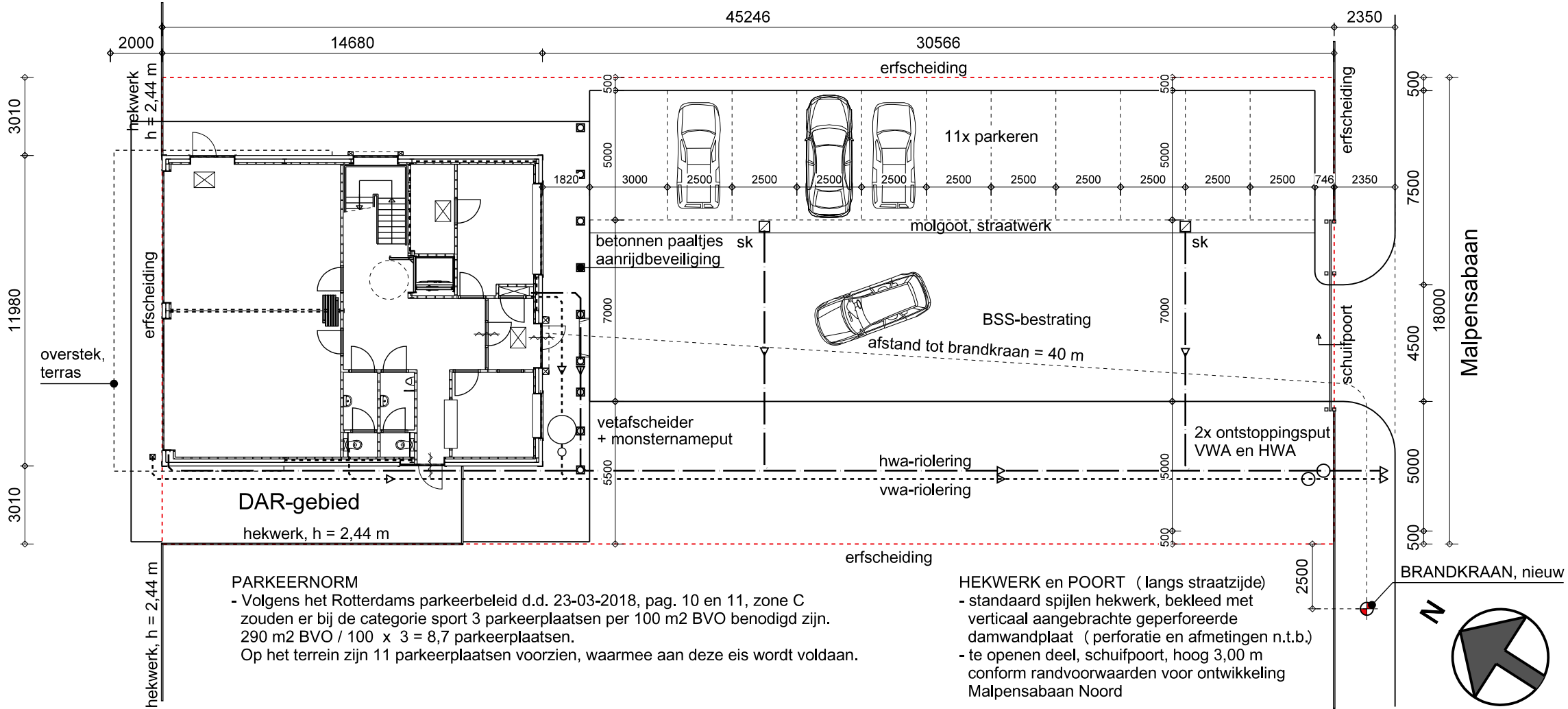
terrein - nieuw - 1: 200
