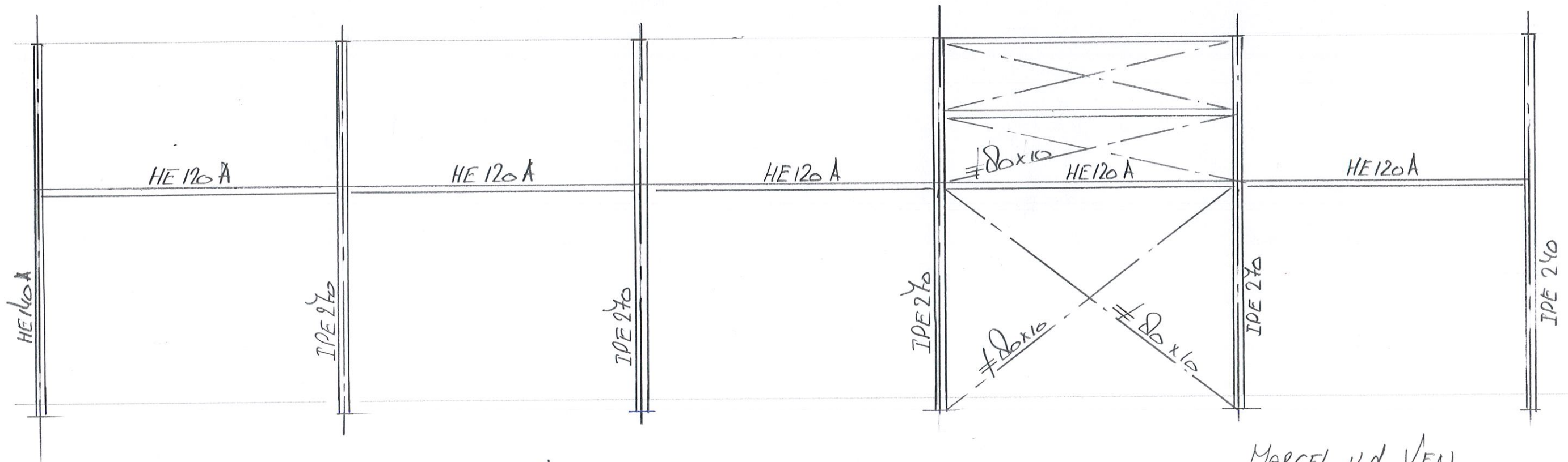
NOORD GEVEL.
