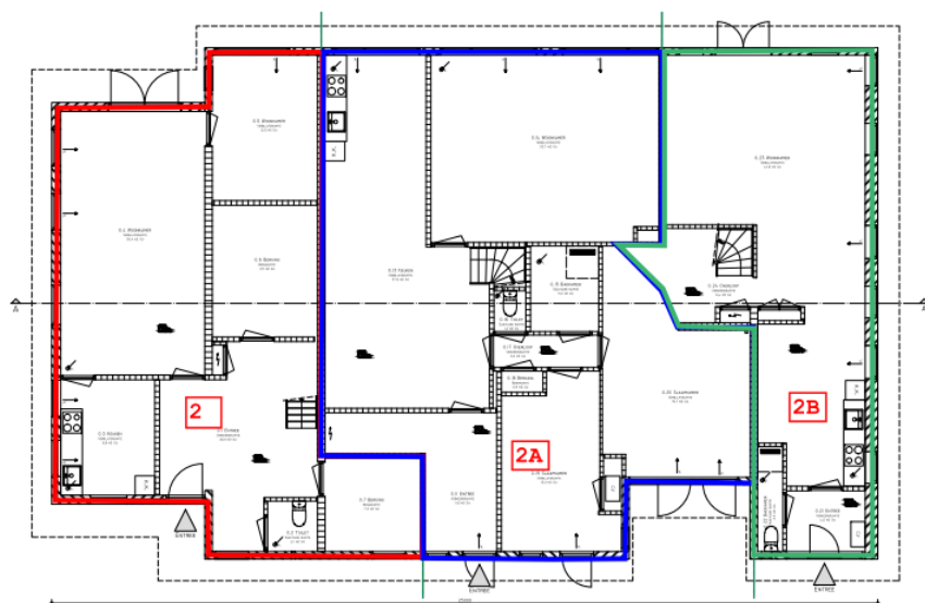
Begane grond
