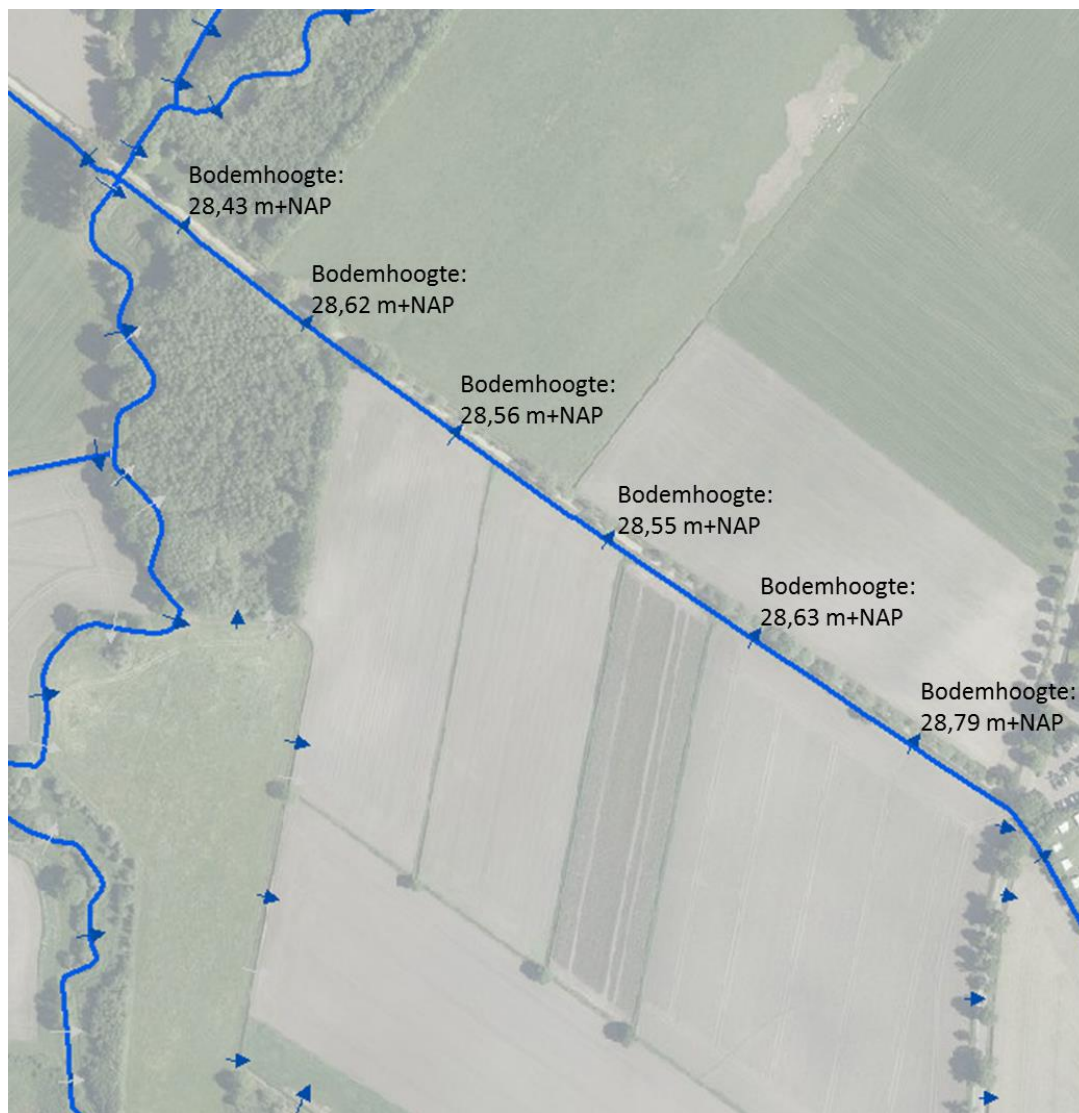
Figuur 41 Bodemhoogtes KS29.
