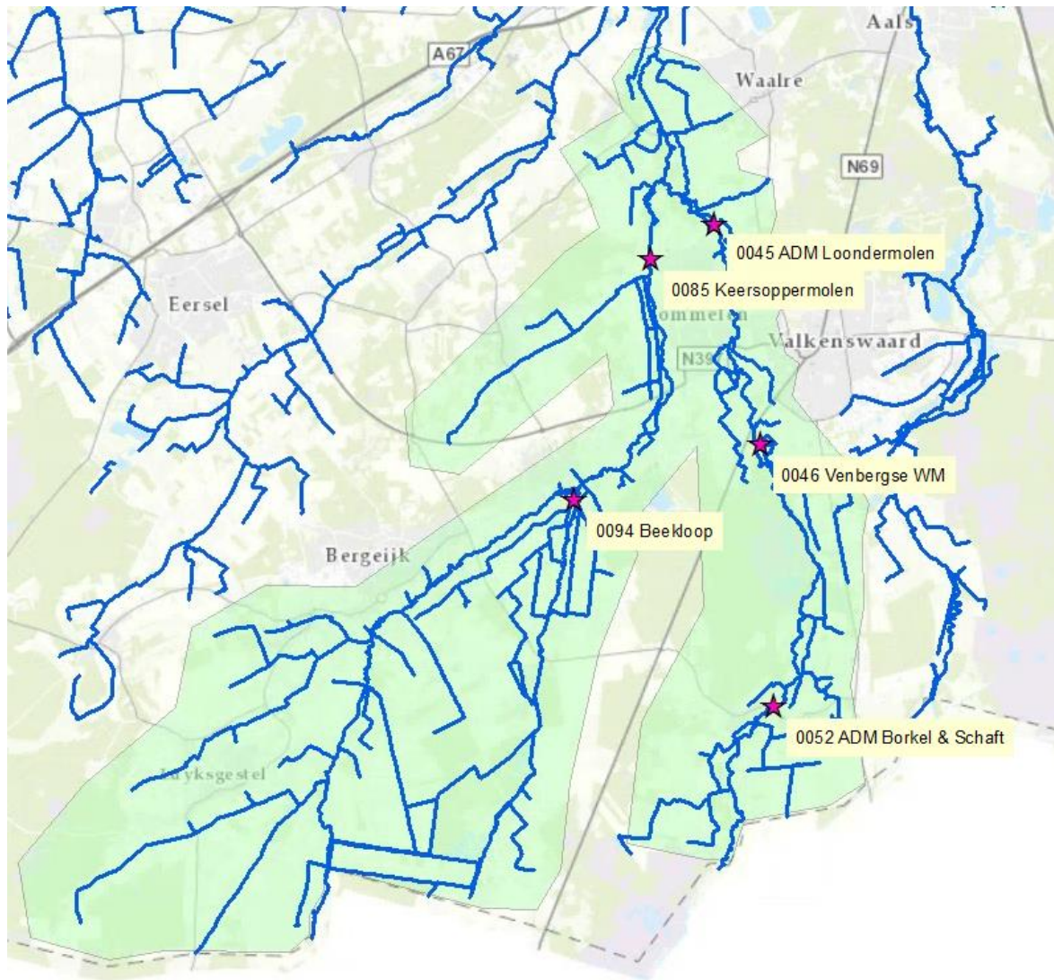
Figuur 3 Meetlocaties gebruikt bij de kalibratie en validatie van het Sobek-model van de Keersop en Dommel bovenstrooms Waalre.
