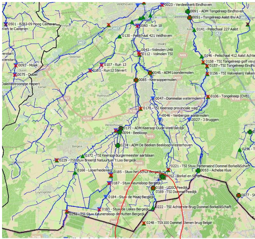
Figuur 3 Overzicht van modelgebied Dommel Vlaanderen.
