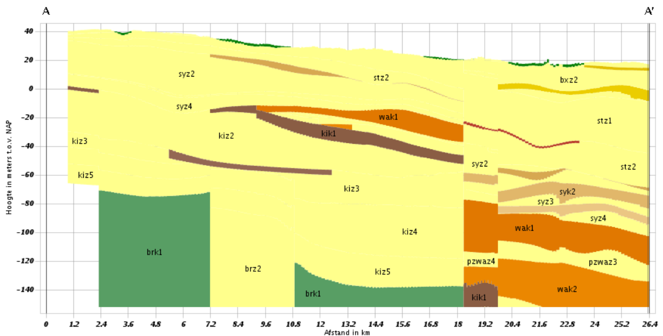
Verticale Doorsnede REGIS II v2.1
