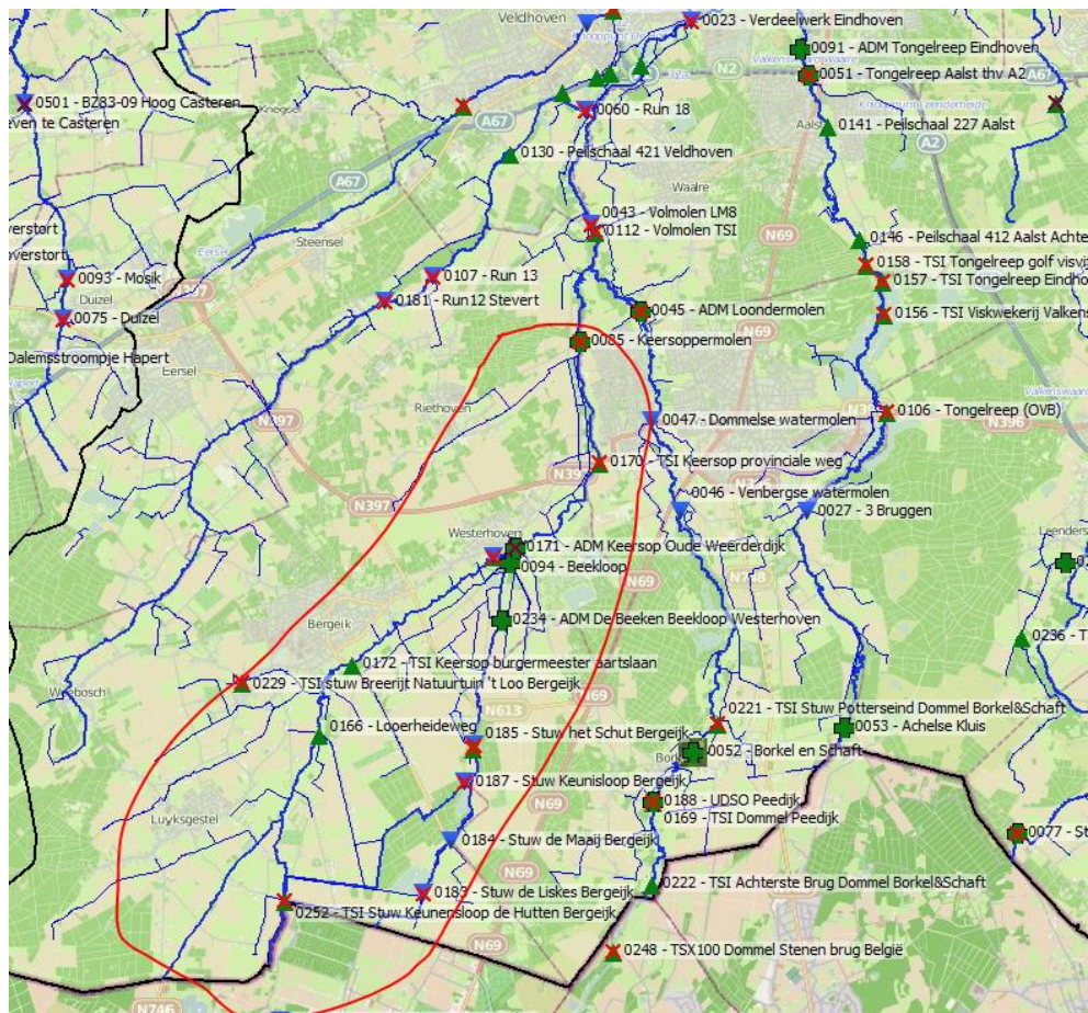
Figuur 2 Overzicht van modelgebied Keersop.
