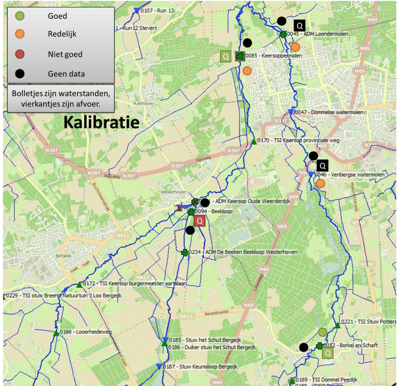
Figuur 4 Overzicht van modelprestaties tijdens kalibratieperiode
