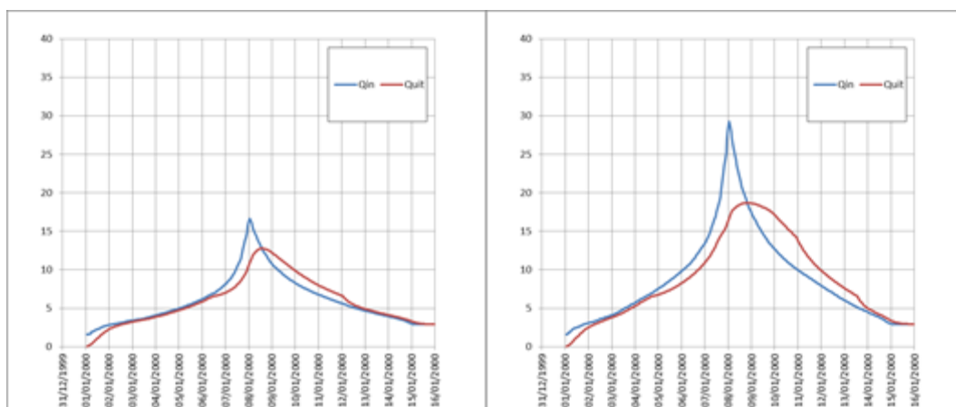
figuur 2 demping afvoergolf stroomgebied in België, links = T10, rechts = T100.
