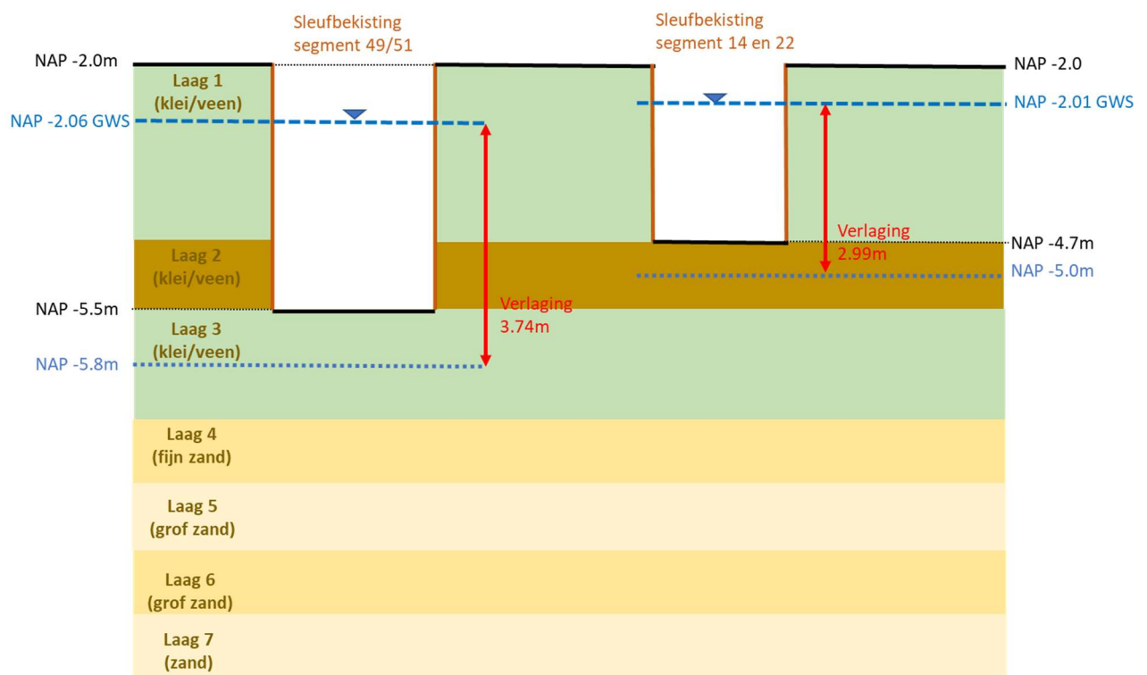
Figuur 2a: Schematische dwarsdoorsnede freatisch pakket met ingreep
