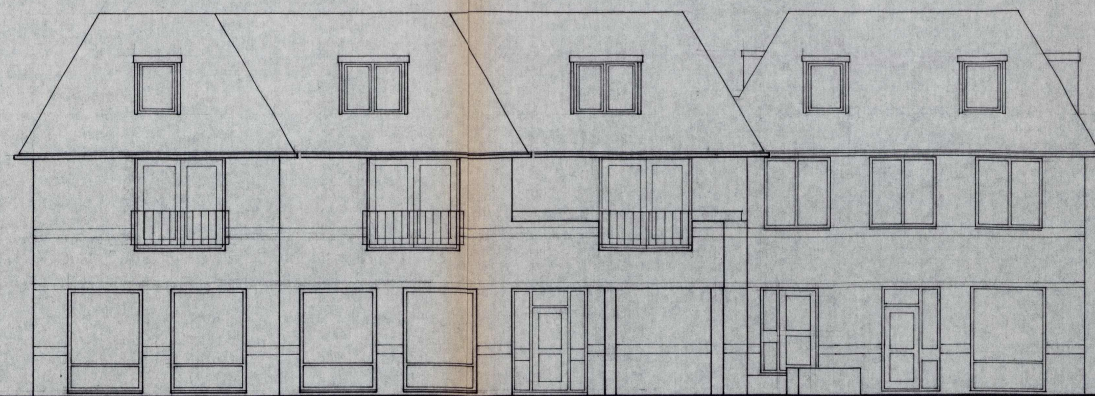
WESTGEVEL
