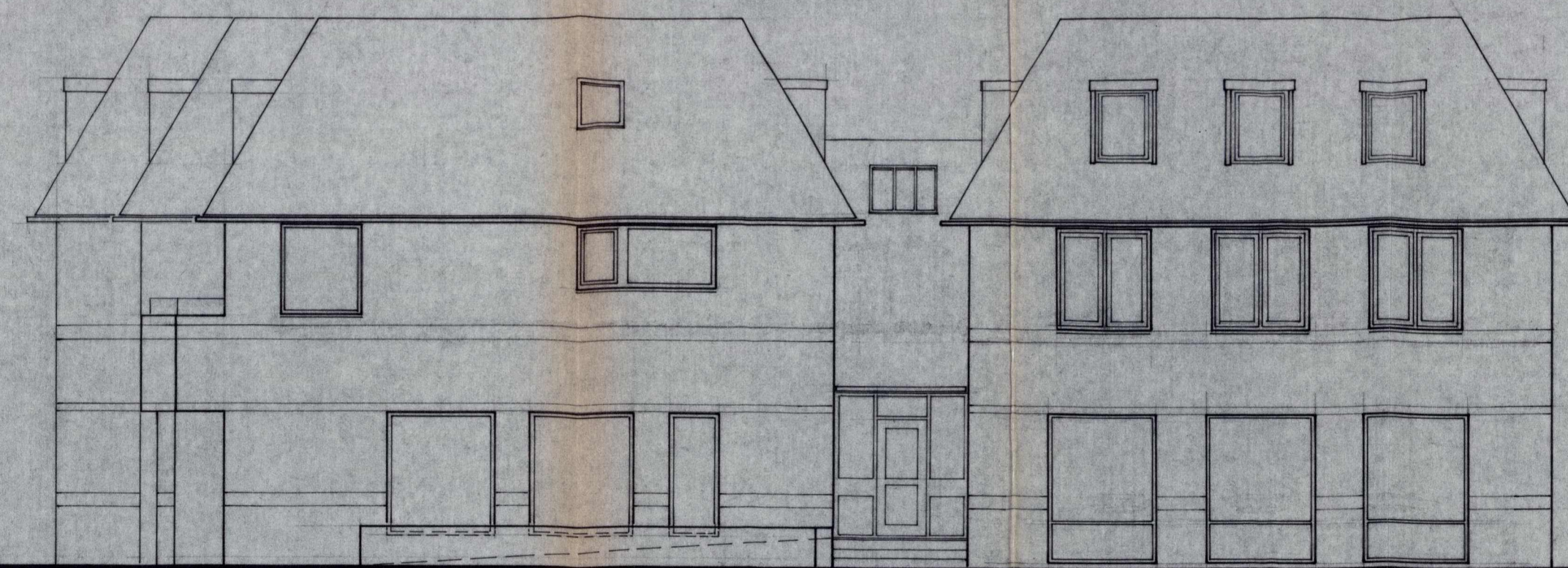
ZUIDGEVEL
