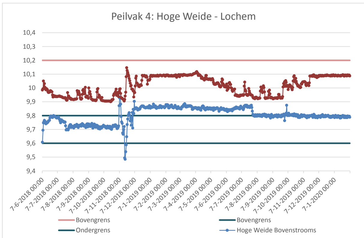
Figuur 18: Toetsing peilen aan meetgegevens.
