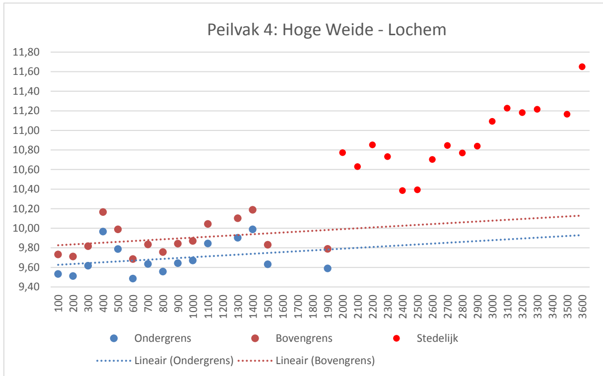
Figuur 19: Maatgevende drooglegging t.o.v. NAP voor stuwpand Hoge Weide-Lochem.
