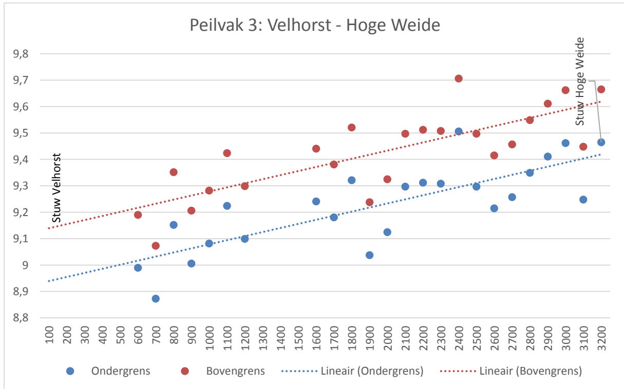
Figuur 15: Maatgevende drooglegging t.o.v. NAP voor stuwpand Velhorst-Hoge Weide.
