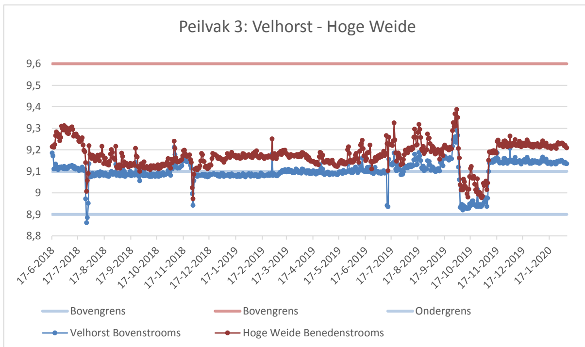
Figuur 16: Toetsing peilen aan meetgegevens.
