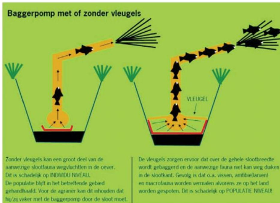
Figuur 1. Met een baggerpomp zonder vleugels wordt het schonen van de sloten (zoals weergegeven in figuur 2 van bijlage 4) uitgevoerd.
