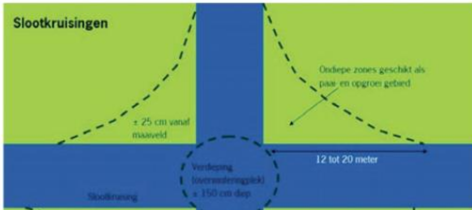
Figuur 2. Sloot 38 (zie figuur 2 bijlage 4) wordt volgens dit figuur geherprofileerd.
