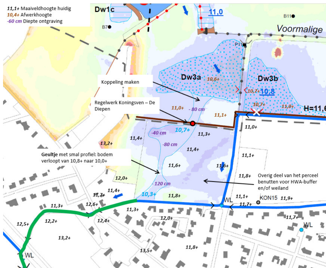
Figuur 9 Koppeling De Diepen – Tielebeek: Variant 3
