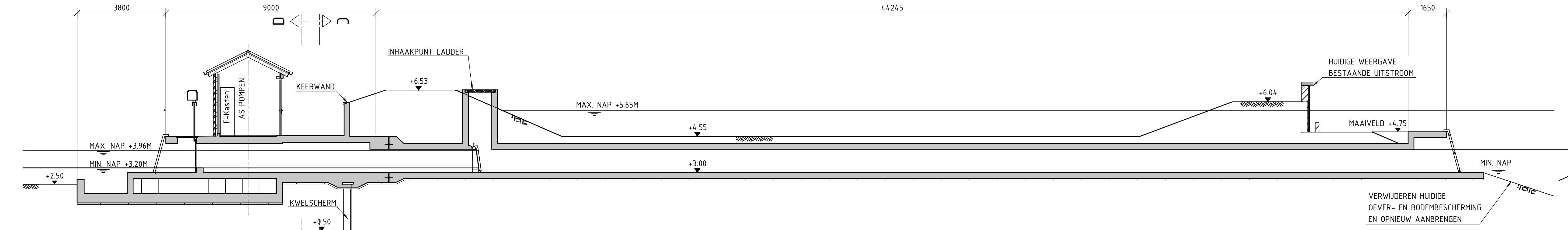
DOORSNEDE A - A SCHAAL 1:100
