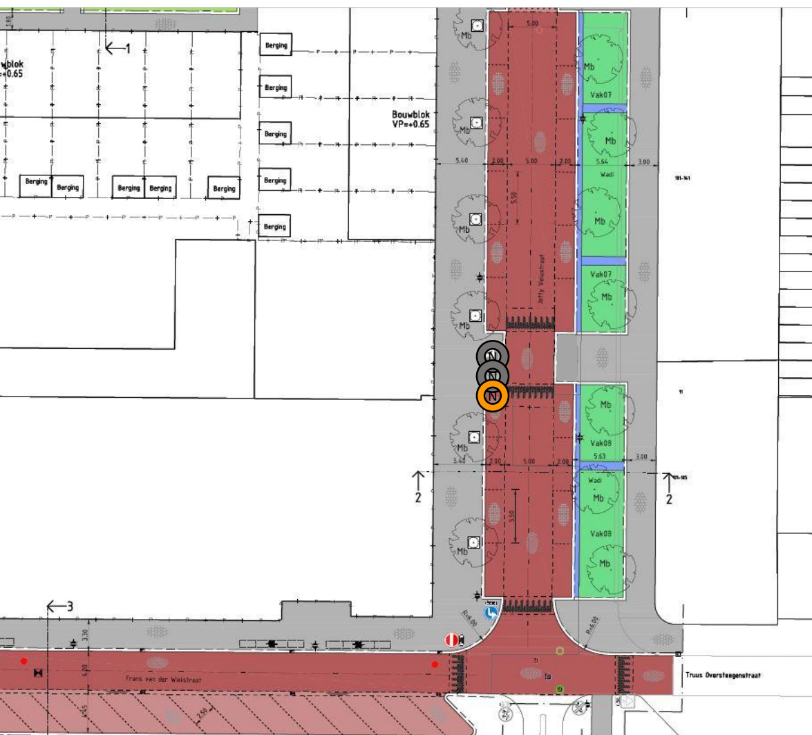
Projectie afvalinzameling in herinrichtingsplan Blok 5
