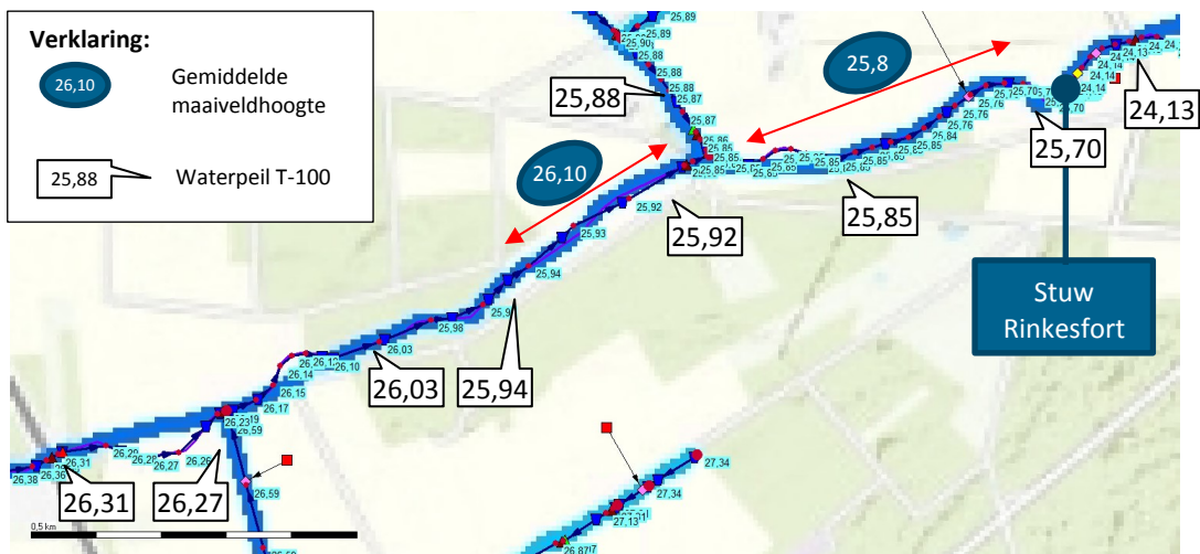
Figuur 4-17: Maximaal peil bij een T100-worst-case-situatie tijdens inzet van de berging (toekomstige situatie).
