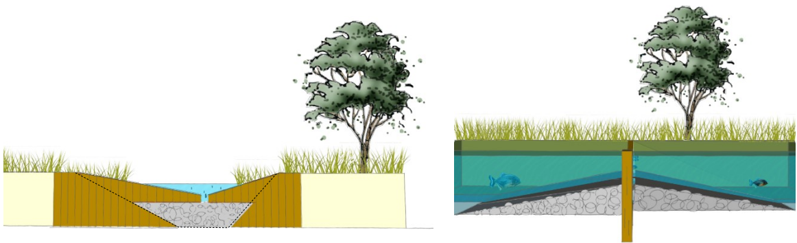
Figuur 4-31: principe cascade
