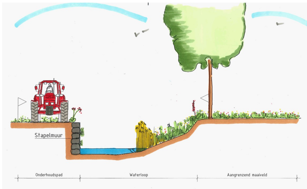
Figuur 4-26: Principeprofiel Kwistbeek benedenloop met eenzijdig stapelmuur dorpskern Baarlo
