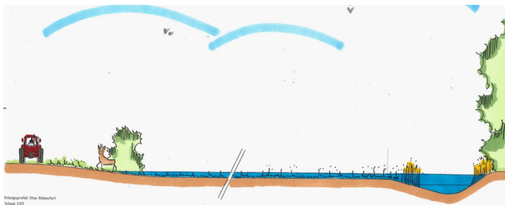
Figuur 4-15: Principeprofiel beekdalberging bovenstrooms stuw Rinkesfort ten tijde van berging
