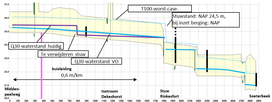
Figuur 4-13: VO-ontwerp met de Q30-zomerwaterstand in de huidige (paarse lijn) en toekomstige situatie (blauwe lijn) en de T100-worst-case-waterstand in de toekomstige situatie bij inzet van de berging.
