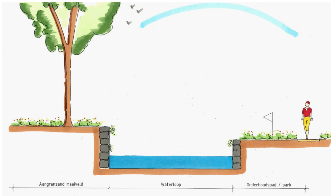
Figuur 4-28: Principeprofiel Kwistbeek benedenloop met tweezijdig stapelmuur bovenstrooms van de Watermolen in Baarlo
