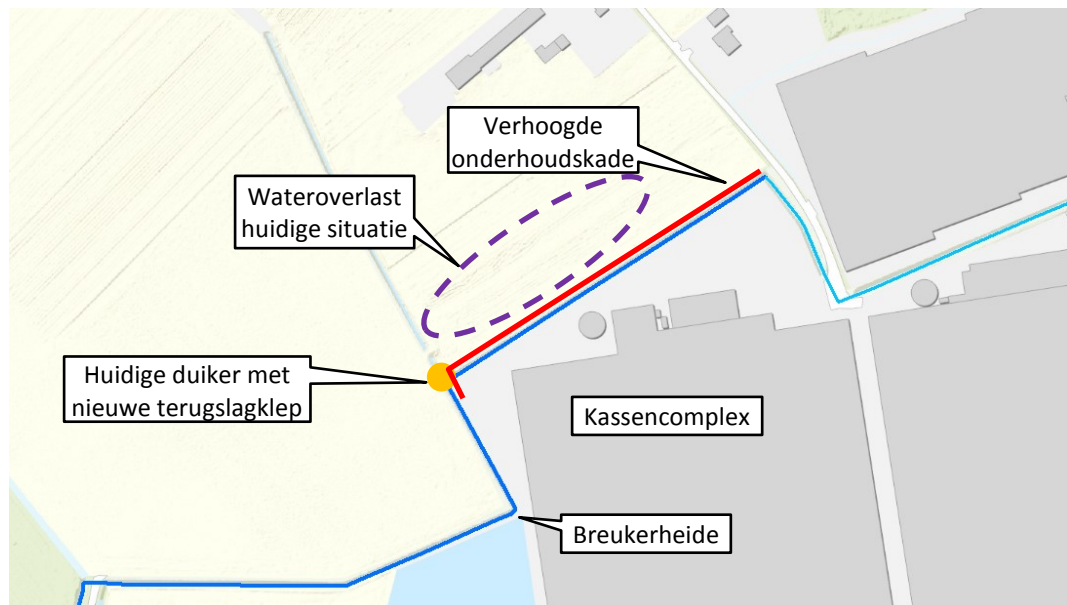
Figuur 4-38: Toekomstige inrichting Breukerheide bij Vlasrooth.
