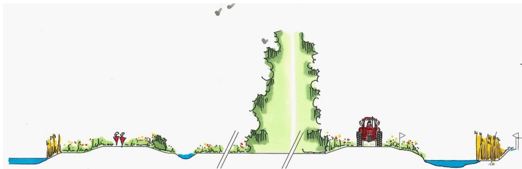
Figuur 4-5: Principedoorsnede overloopgebied de Baendj
