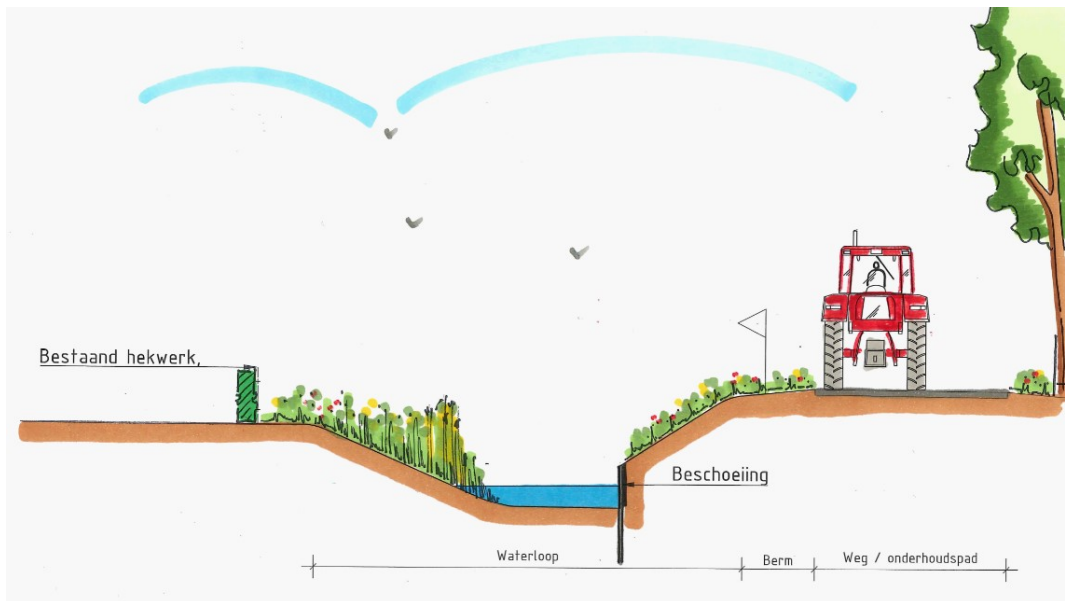
Figuur 4-25: Principeprofiel Kwistbeek benedenloop eenzijdig beschoeiing, ter hoogte Soeterbeek
