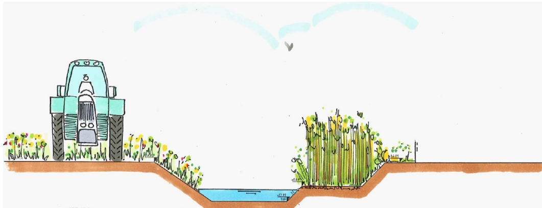
Figuur 4-3: Principeprofiel Plasdraszone (accoladeprofiel)
