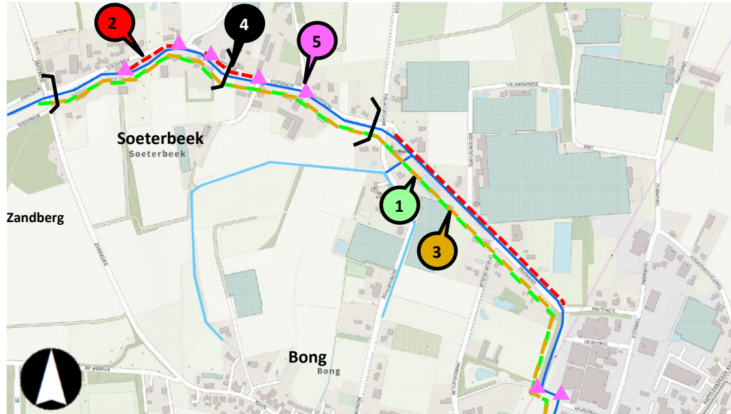
Figuur 4-21: Overzicht maatregelen Benedenloop, deel 1
