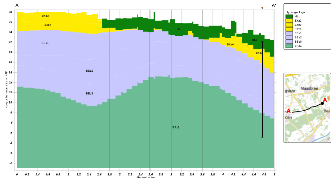
Figuur 2-4: Doorsnede van de bodembouw.
