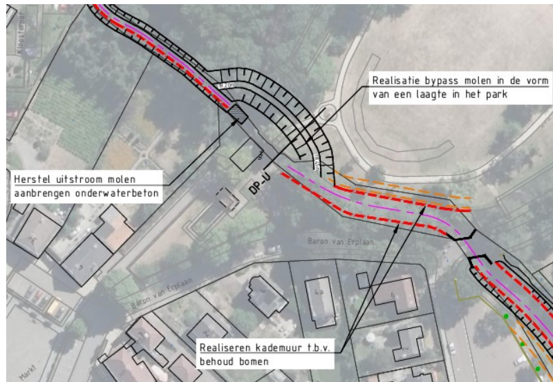
Figuur 4-34: bovenaanzicht bypass molen
