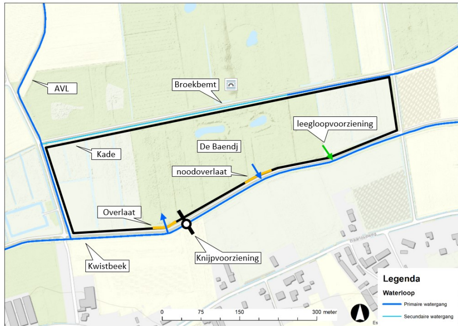
Figuur 4-4: Inrichtingsprincipe overloopgebied de Baendj
