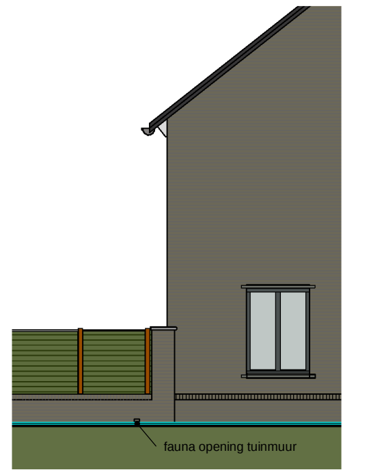
aanzicht blok 5
