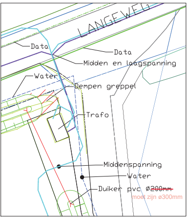
Nieuwe situatie bij trafoverdeelstation kruising Polderweg & Langeweg, Kruisland. Schaal 1:100
