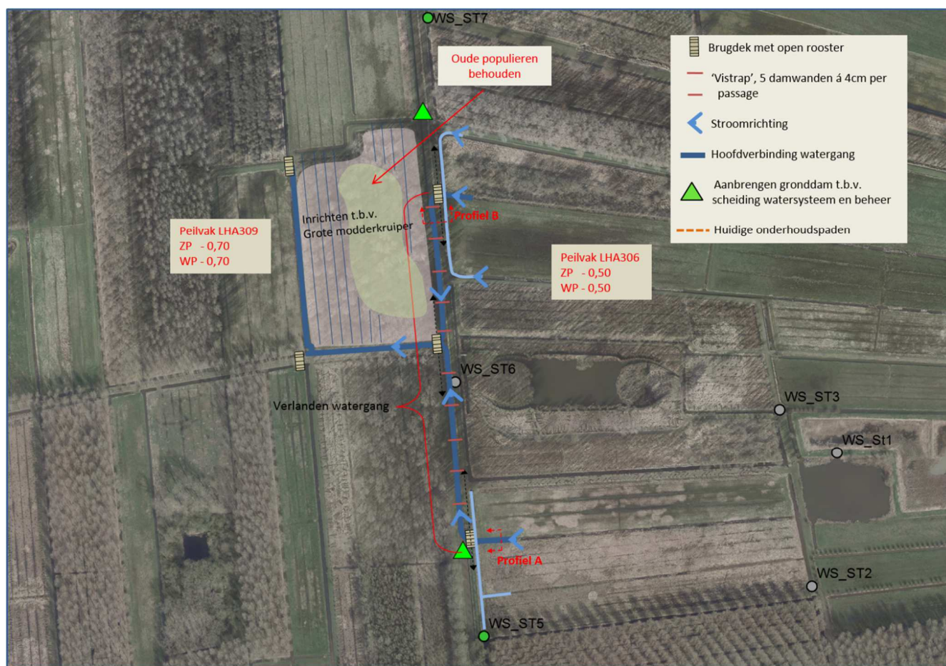
Figuur 3-2 Schetsontwerp van de verbinding voor de Grote modderkruiper
