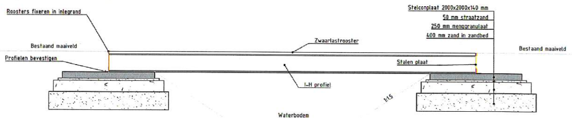
Figuur 13 Principedetail van een roosterbrug die wordt aangebracht om de bestaande onderhoudsroutes intact te laten.
