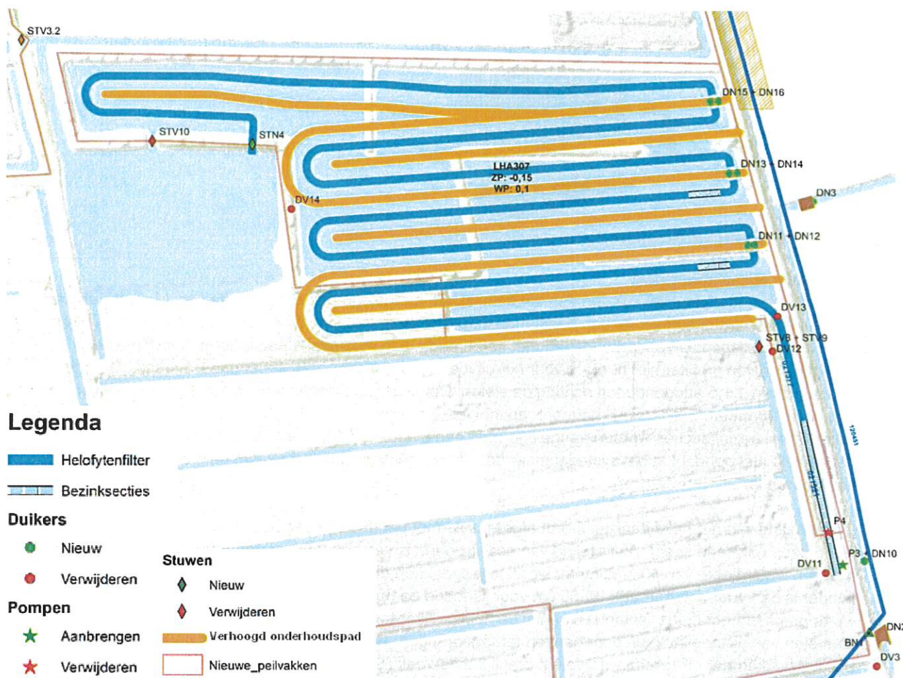
Figuur 15 overzicht maatregelen aan waterstaatswerken Helofytenfilter.
