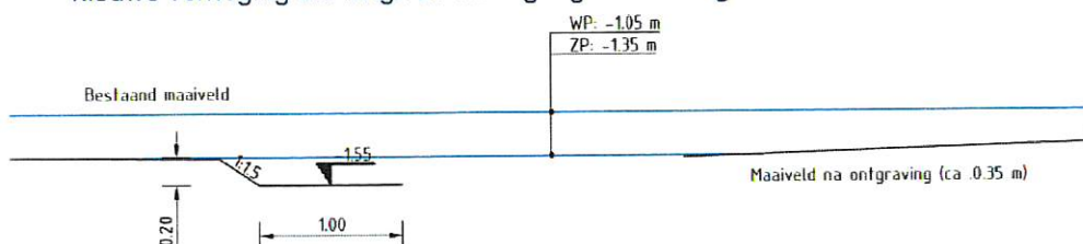
Figuur 21 Aangepast profiel met een natuurvriendelijke oever voor de bestaande noord- zuidgeoriënteerde watergangen.
