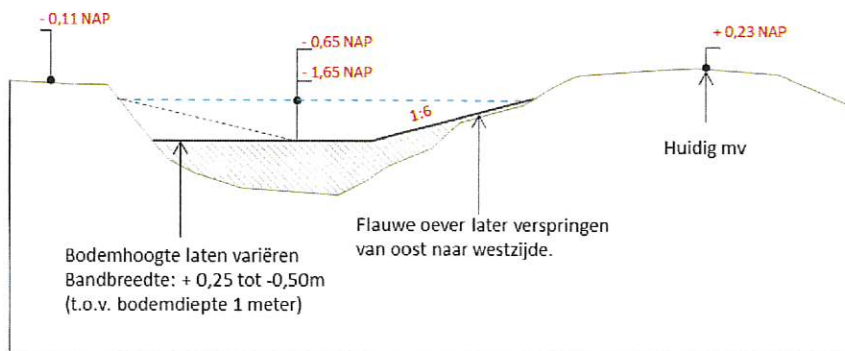
Figuur 9 Principeprofiel van de inrichting voor Krabbescheervegetaties.
