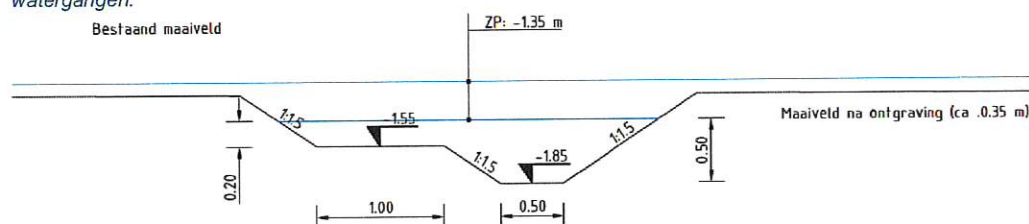
Figuur 22 Profiel nieuwe watergang ten bate van de Grote modderkruiper.
