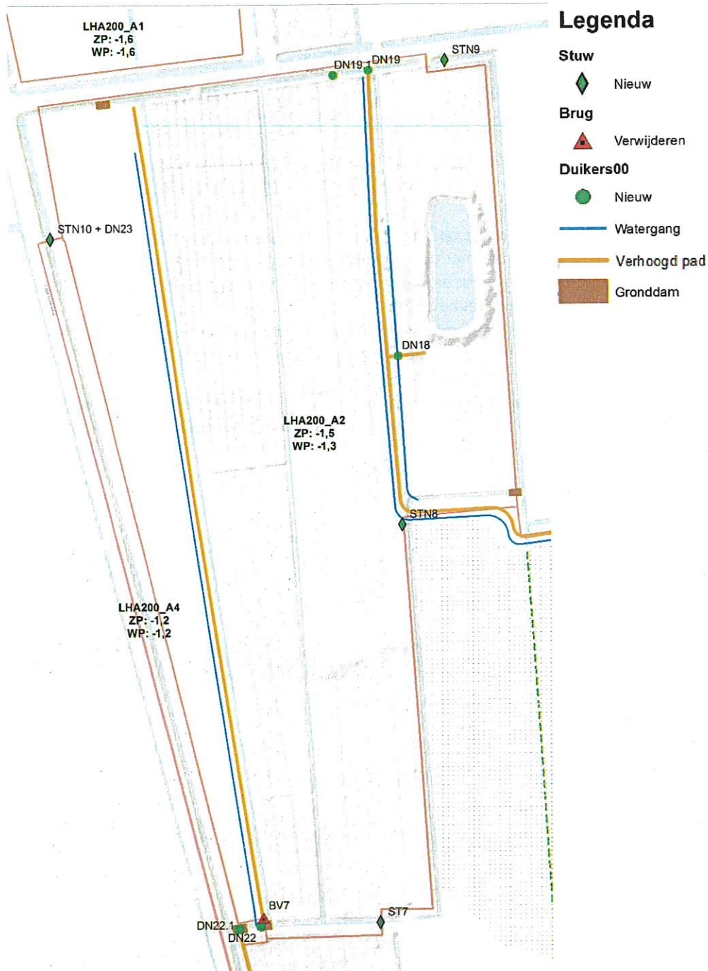
Figuur 24 Overzicht van maatregelen aan waterstaatswerken.
