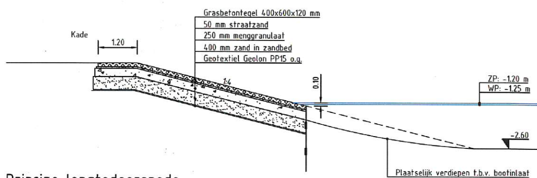
Principe lengtedoorsnede bootinlaathelling
