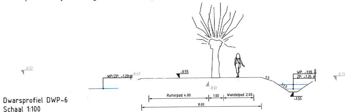
Figuur 18 Profiel van de zuidelijke verhoging waarop zowel een wandel- als ruiterspad is gesitueerd.
