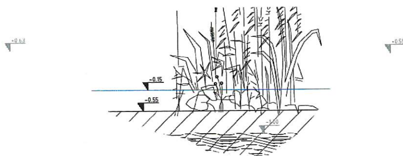
Figuur 16 Verondiepen van de aanvoersloot t.b.v. het helofytenfilter.
