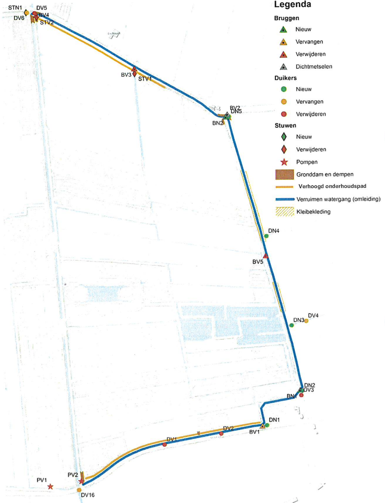
Figuur 4 Overzicht van maatregelen aan waterstaatwerken
