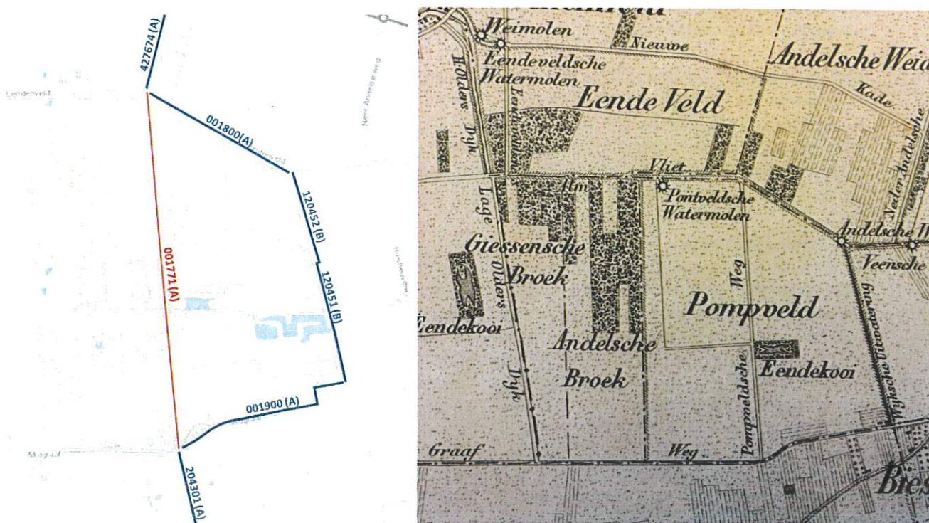
Figuur 6 (Links) Overzicht van de watergangen die worden verruimd ten bate van de omleiding. (Rechts) Een historische kaart die laat zien dat op de locatie waar die nieuwe hoofdwatergang is gesitueerd, vroeger ook de Wyksche Uitwatering is gelegen.
