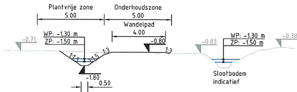
Figuur 25 profiel van verhoogd onderhoudspad en watergang zoals omschreven bij maatregel 6.1. en 6.2.
