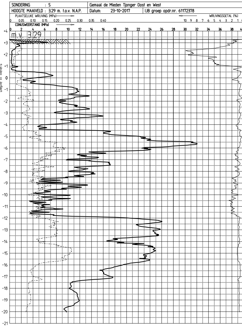
SONDERING 5 SCHAAL 1:200
