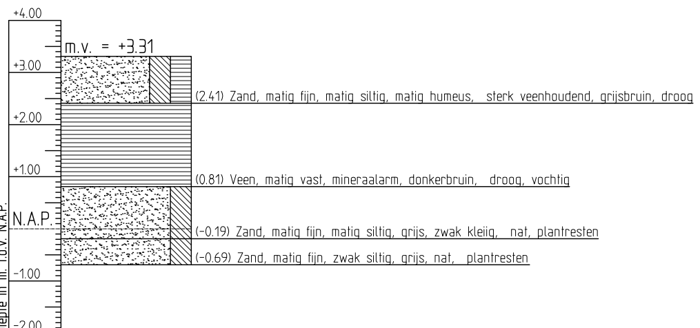
BORING C SCHAAL 1:100
