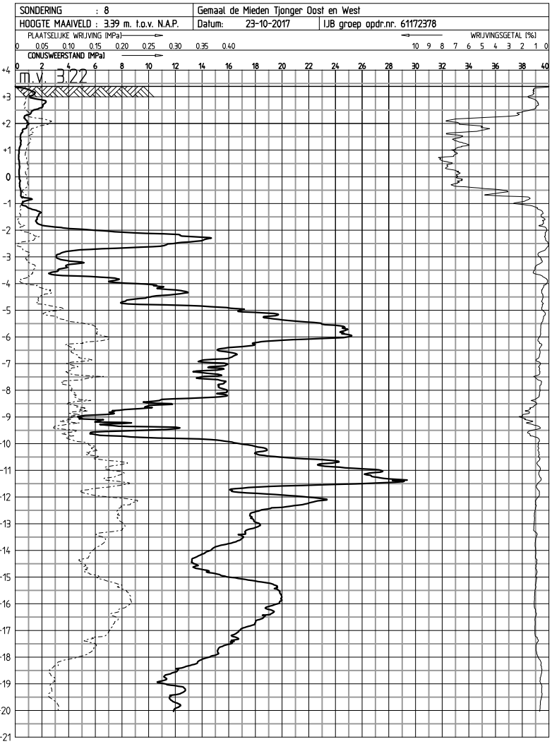
SONDERING 8 SCHAAL 1:200
