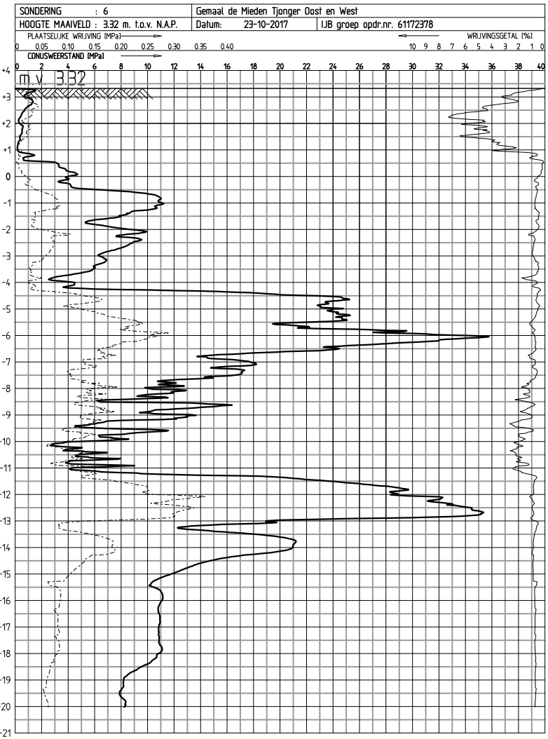
SONDERING 6 SCHAAL 1:200
