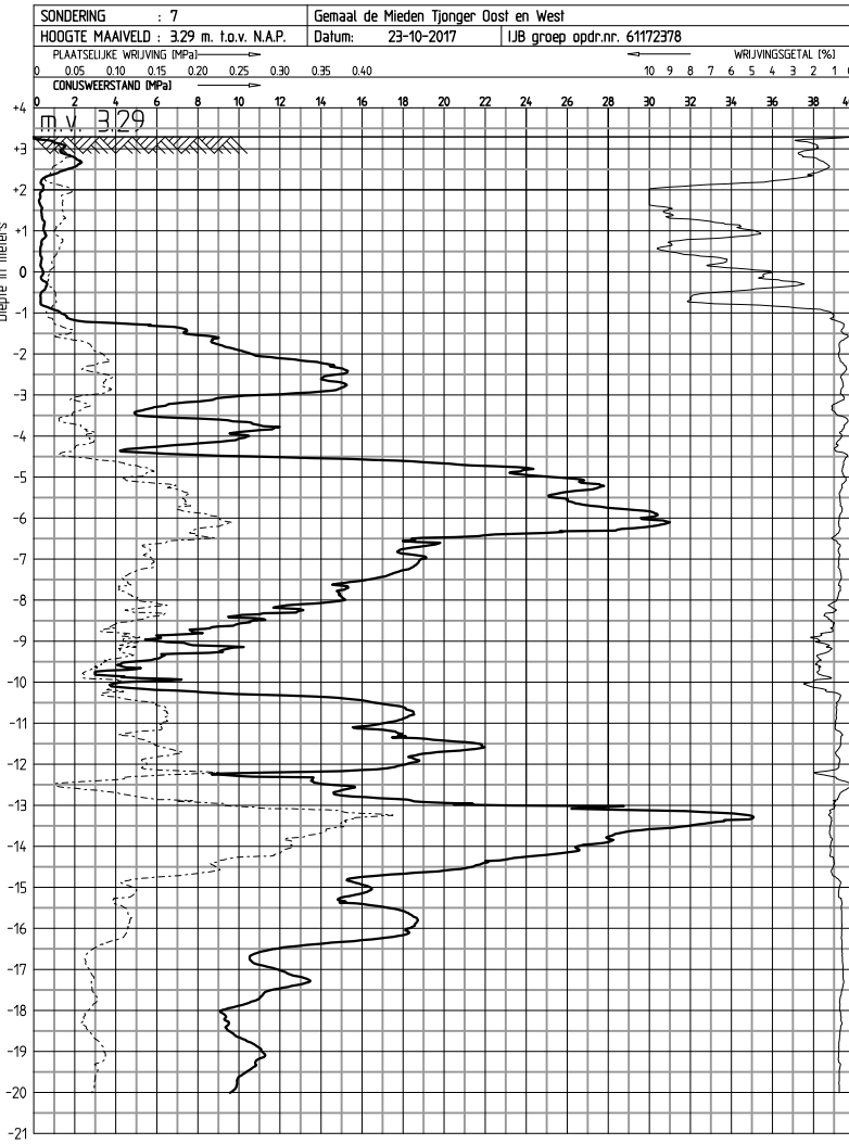
SONDERING 7 SCHAAL 1:200
