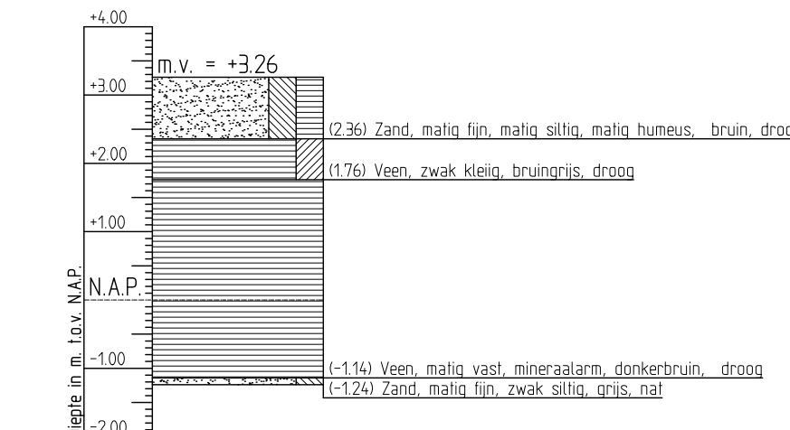
BORING D SCHAAL 1:100
